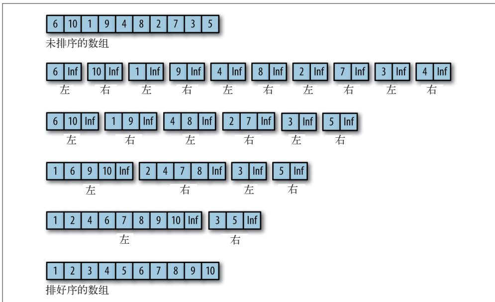
图 12-4：自底向上的归并排序算法
