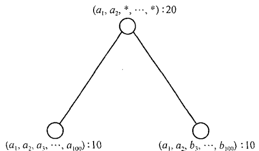
图 5.2 形成闭立方体的格的 3 个闭单元
