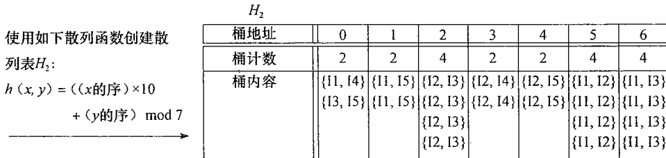
图 6.5 候选 2 项集的散列表 H_2 。该散列表在由 C_1 确定 L_1 时通过扫描表 6.1 的事务数据库产生。如果最小支持度为 3，则桶 0、1、3 和 4 中的项集不可能是频繁的，因此它们不包含在 C_2 中
