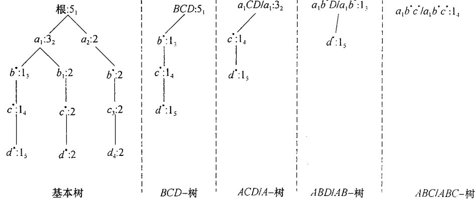
图 5.11 聚集阶段一：处理基本树的最左分支
