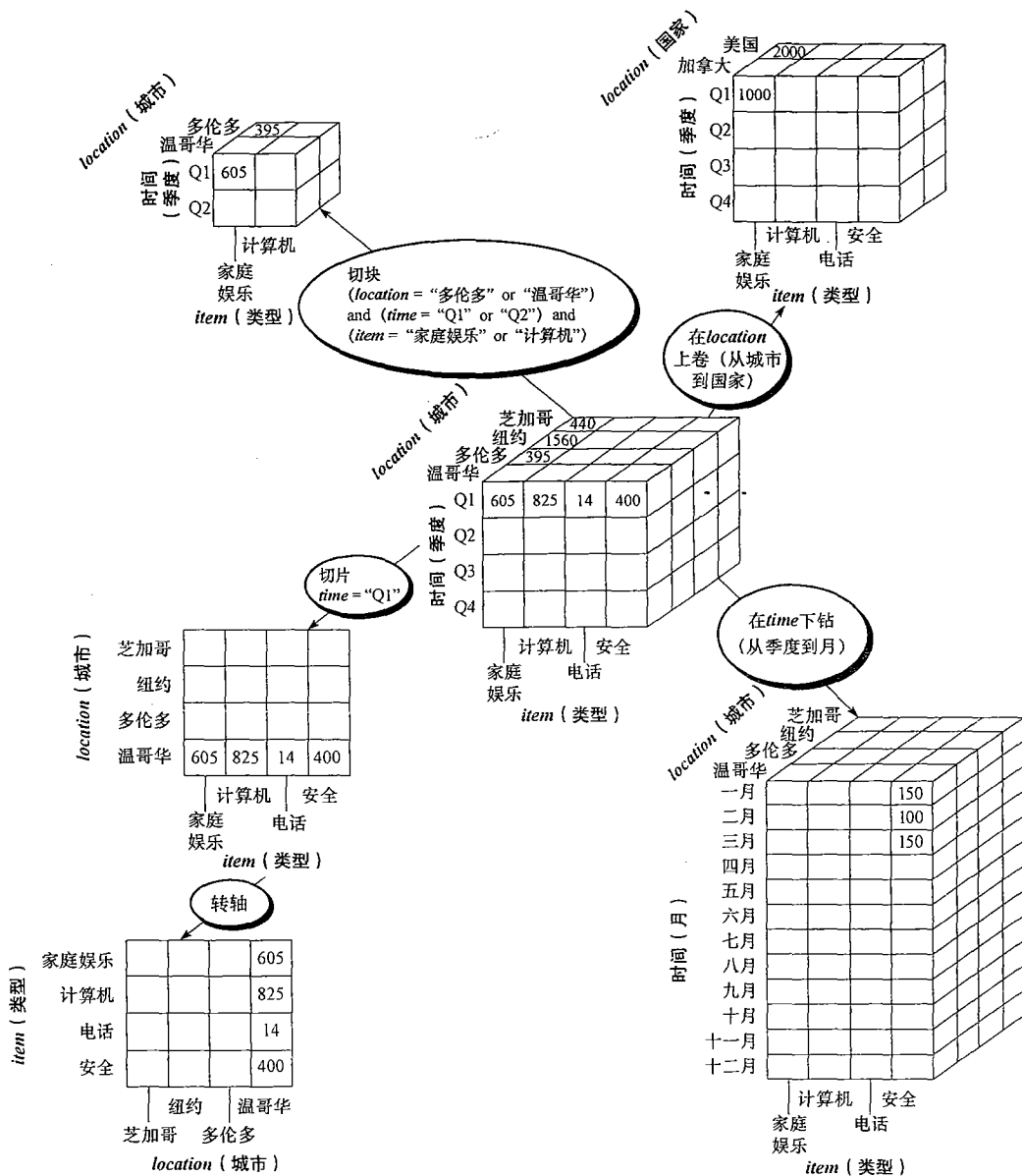
图 4.12 多维数据上的典型 OLAP 操作的例子
