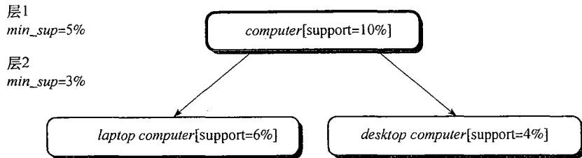
图 7.4 具有递减支持度的多层挖掘
