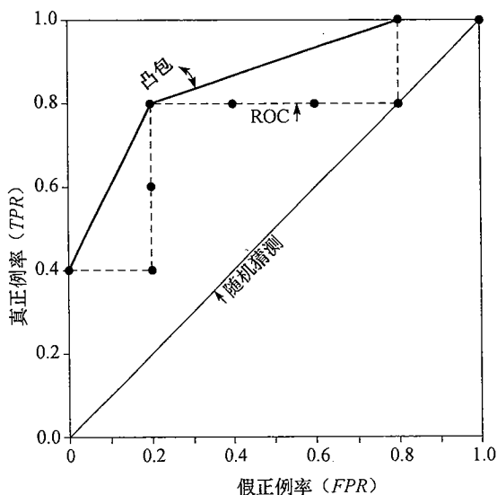
图 8.19 图 8.18 的数据的 ROC 曲线
