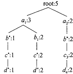
图 5.10 压缩的基本表的星树
