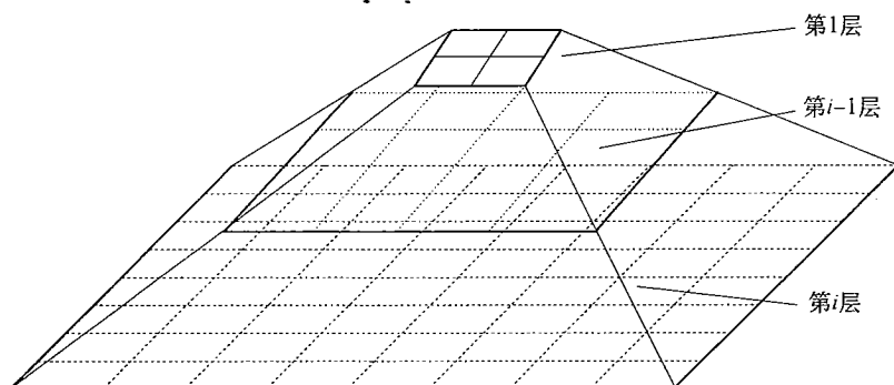
图 10.19 STING 聚类的层次结构
