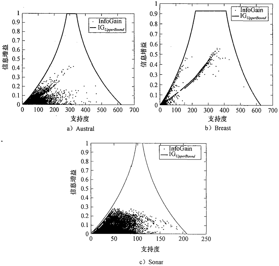
图 9.12 3 个 UCI 数据集的模式频度（支持度）与信息增益。还显示了信息增益的理论上界 ( IG_{UpperBound} )。取自 Cheng、Yan、Han 和 Hsu [CYHH07]
