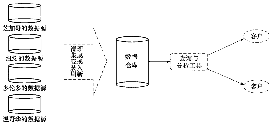
图 1.6 AllElectronics 数据仓库的典型框架
