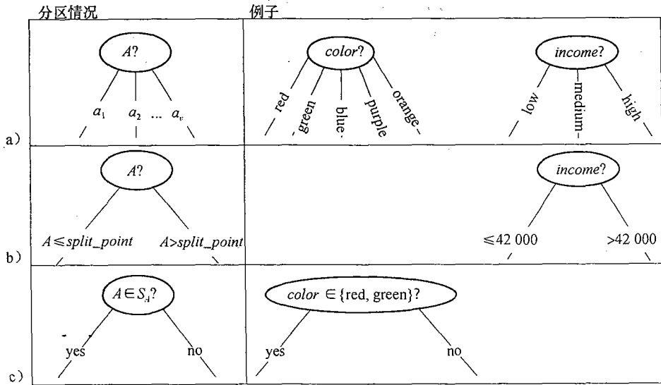
图 8.4 根据分裂准则划分元组的三种可能性，每个都给出了例子。设 A 是分裂属性：a) 如果 A 是离散值的，则对 A 的每个已知值产生一个分枝；b) 如果 A 是连续值的，则产生两个分枝，分别对应于 A \leq split\_point 和 A > split\_point ；c) 如果 A 是离散值的，并且必须产生二叉树，则测试形如 A \in S_A ，其中 S_A 是 A 的分裂子集
