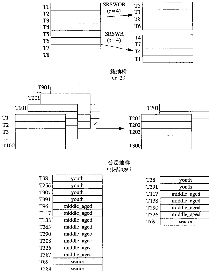
图 3.9 抽样可以用于数据归约
