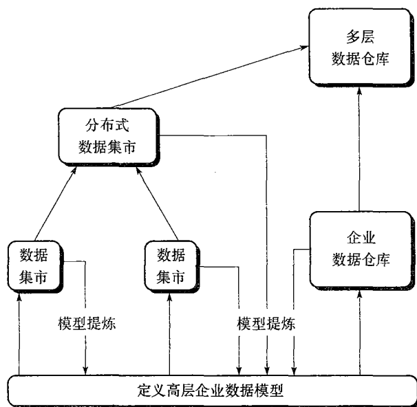
图 4.2 数据仓库开发的推荐方法
