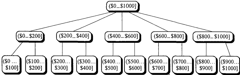
图 4.11 price 的概念分层
