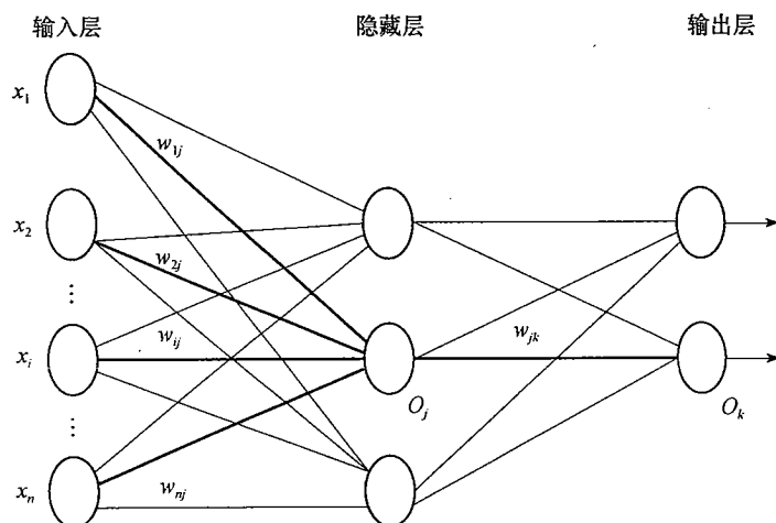
图 9.2 一个多层前馈神经网络
