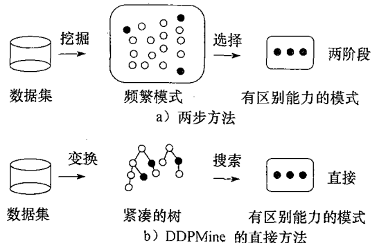
图 9.13 基于频繁模式分类的框架
