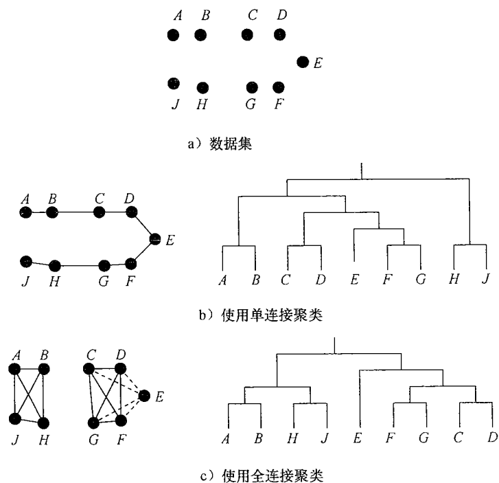
图 10.8 使用单连接聚类和全连接聚类
