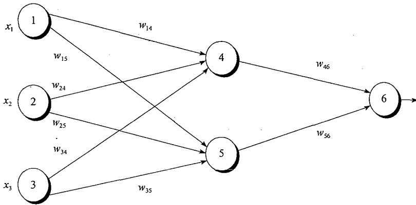
图 9.5 多层前馈神经网络的一个例子
