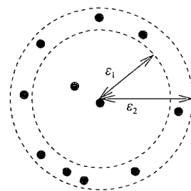
图 10.18 DBSCAN 和 OPTICS 中密度估计的微妙变化。邻域半径从 \epsilon_1 稍增加到 \epsilon_2 导致高得多的密度
