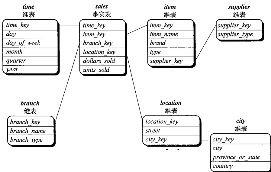
图 4.7 sales 数据仓库的雪花模式
