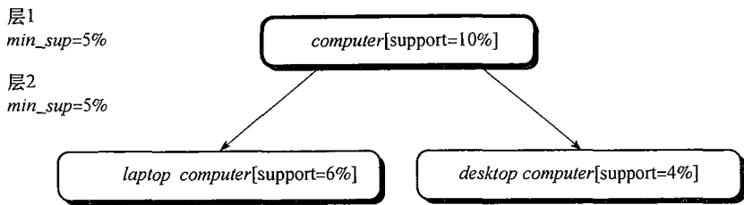
图 7.3 具有一致支持度的多层挖掘
