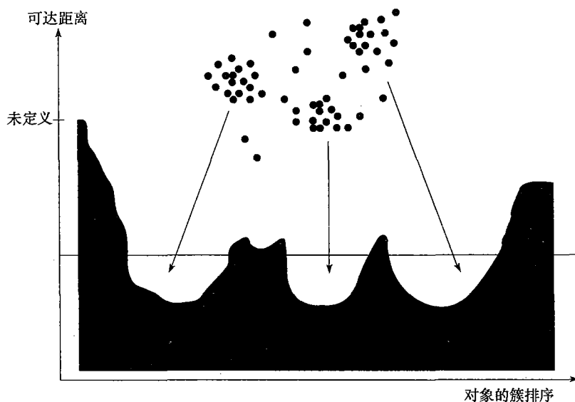
图 10.17 OPTICS 中的簇次序。取自 Ankerst、Breunig、Kriegel 和 Sander[ABKS99]
