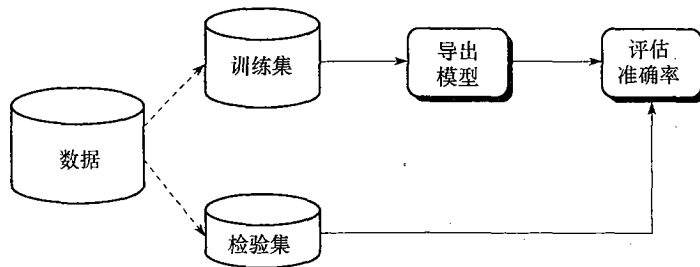
图 8.17 用保持方法估计准确率
