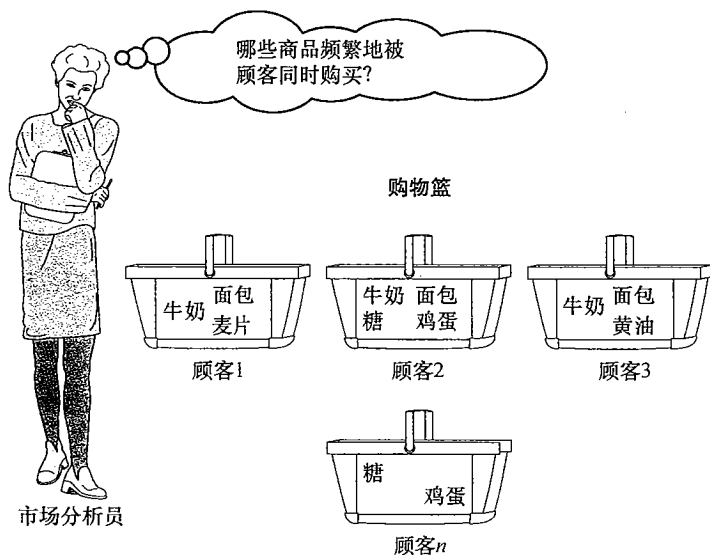
图 6.1 购物篮分析
