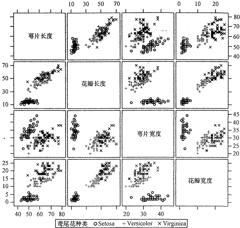
图 2.15 鸢尾花数据集使用散点图矩阵可视化。资料来源： http://support.sas.com/documentation/cdl/en/grstatproc/61948/HTML/default/images/gsgsamat.gif
