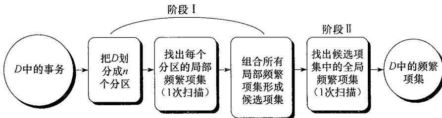
图 6.6 通过划分挖掘
