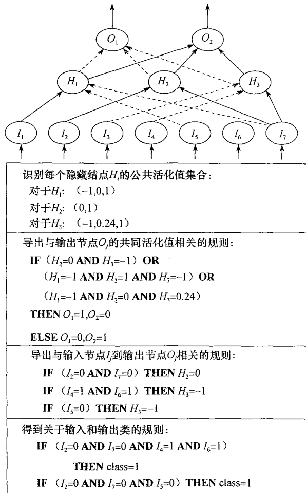
图9.6 可以从训练神经网络提取规则。取自 Lu、Setiono 和 Liu [LSL95]
