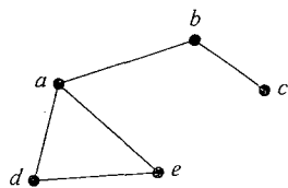
■ 图 11.13 图 G ，其中顶点 c ， d 和 e 都是外围顶点
