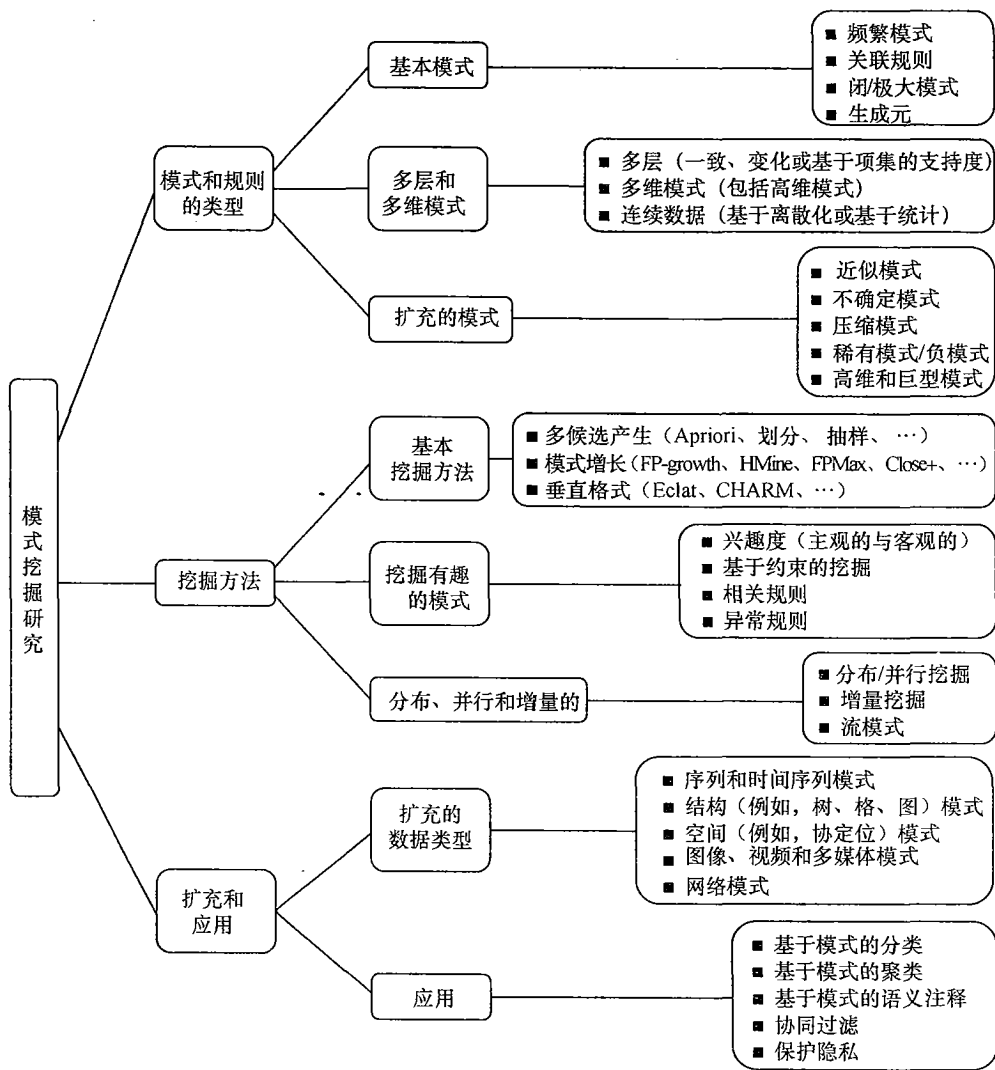
图 7.1 模式挖掘研究的一般路线图
