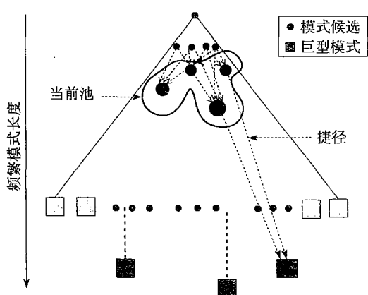
图 7.8 模式树遍历: 候选取自一个模式池, 这导致模式空间通往巨型模式的捷径
