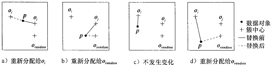
图 10.4 k -中心点聚类代价函数的 4 种情况
