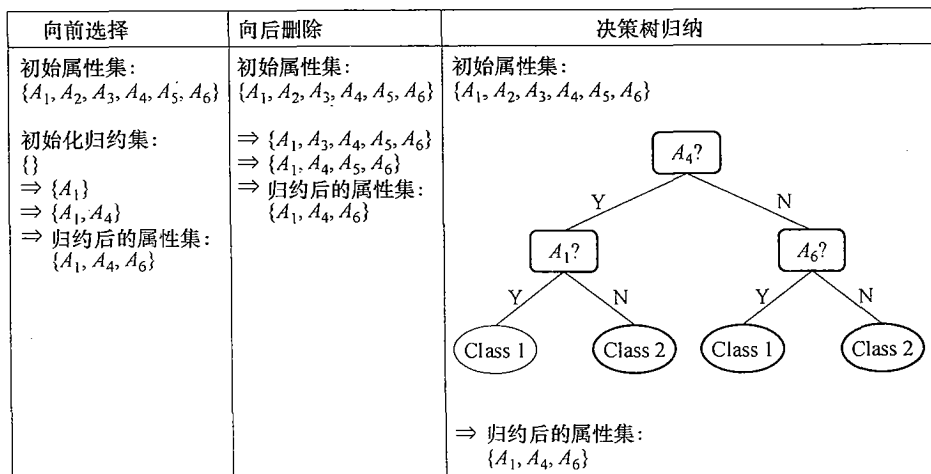
图 3.6 属性子集选择的贪心（启发式）方法
