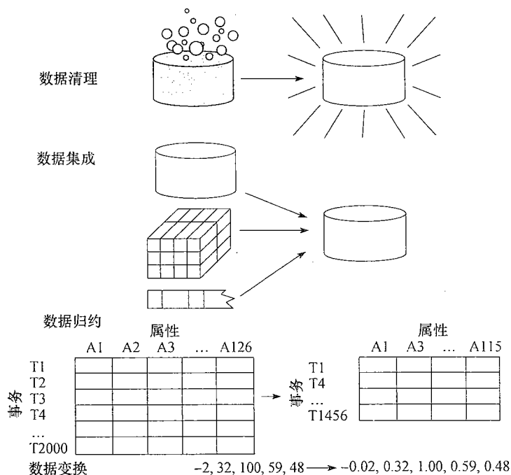
图 3.1 数据预处理的形式
