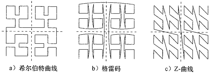
图 2.11 一些频繁使用的二维空间填充曲线
