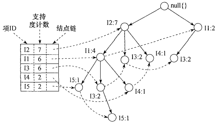
图 6.7 存放压缩的频繁模式信息的 FP 树
