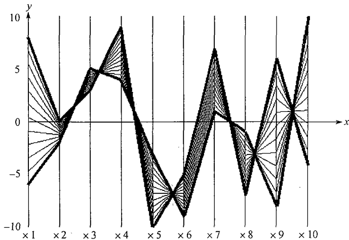
图 2.16 使用平行坐标可视化。资料来源： www.stat.columbia.edu/cook/movabletype/mlm/mdg1.png
