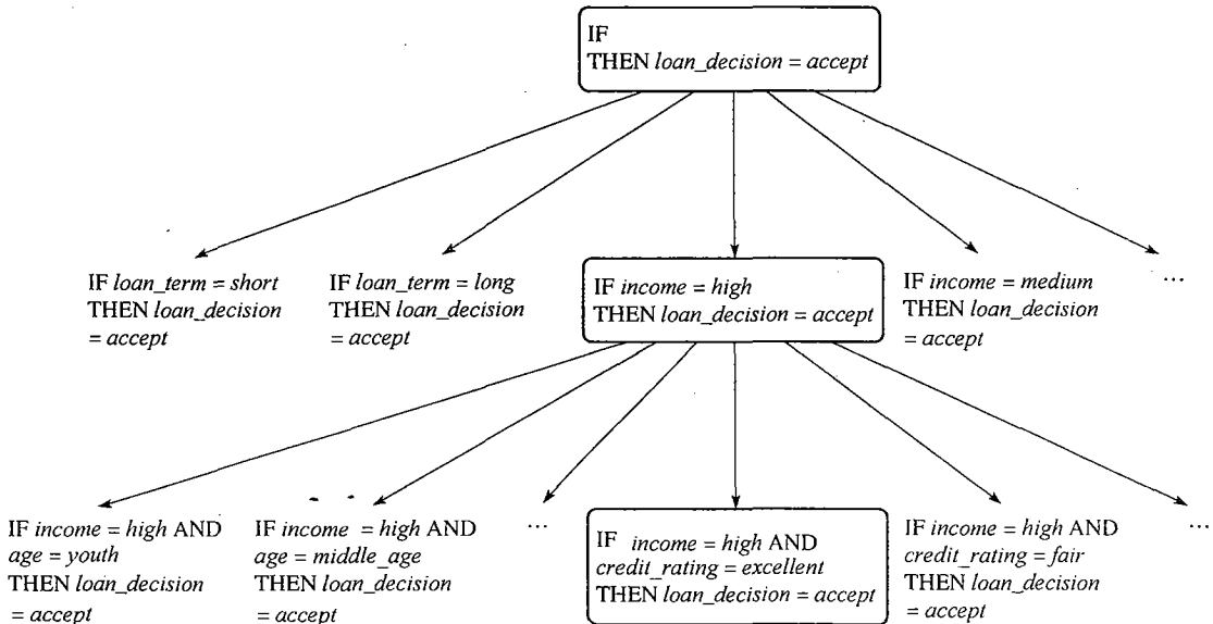
图 8.11 规则空间从一般到特殊搜索
