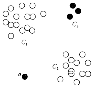
图 12.12 小簇中的离群点
