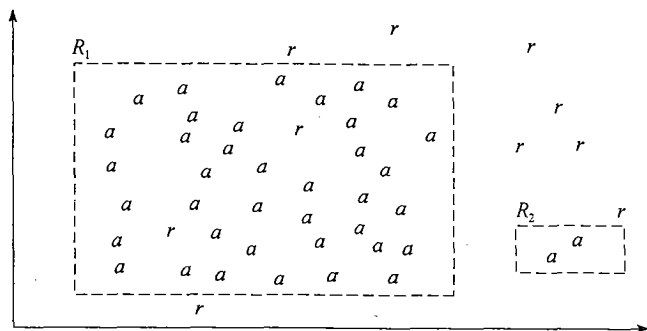
图 8.12 loan\_decision = accept 类的规则，显示 accept(a) 和 reject(r) 元组
