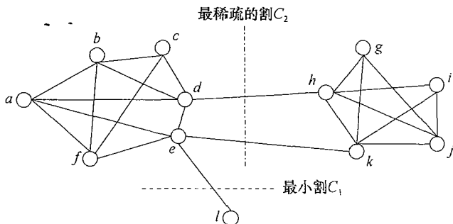
图 11.14 图 G 和它的两个割
