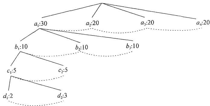
图 5.9 基本方体树的片段
