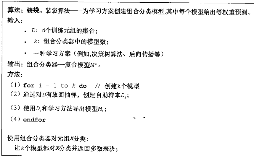
图 8.23 装袋
