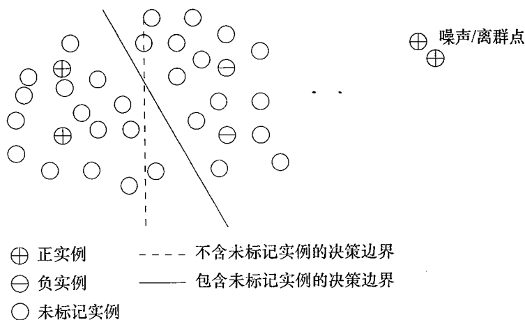
图 1.12 半监督学习
