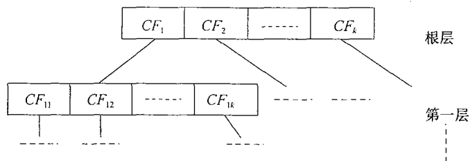
图 10.9 CF-树结构
