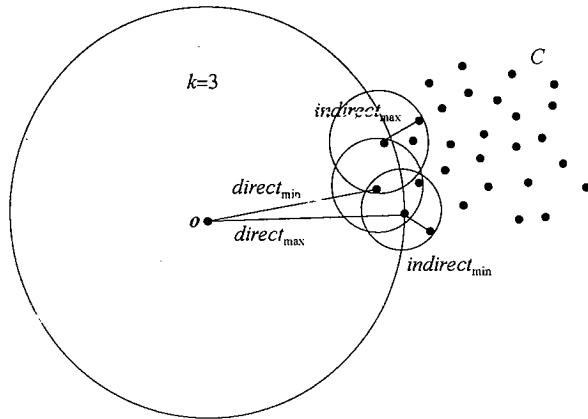
图 12.9 LOF(o) 的性质
