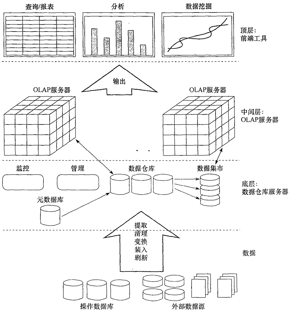
图 4.1 三层数据仓库结构
