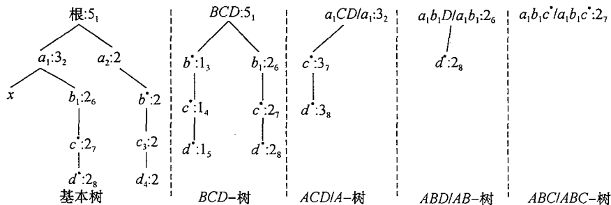
图 5.12 聚集阶段二：处理基本树的第二个分支
