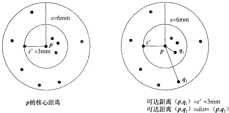
图 10.16 OPTICS 的术语。取自 Ankerst、Breunig、Kriegel 和 Sander [ABKS99]
