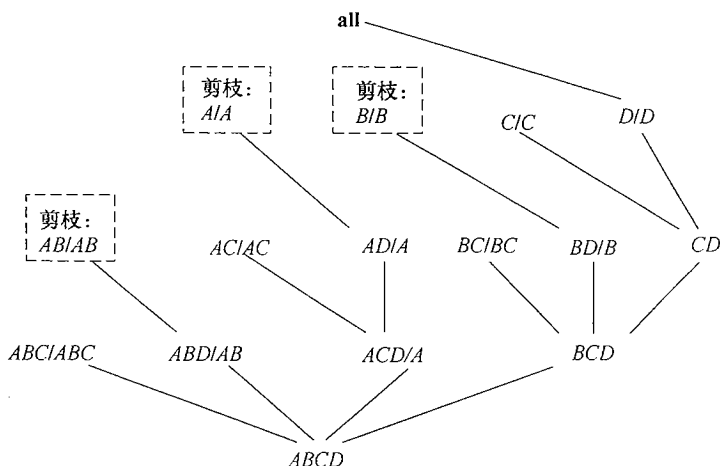
图 5.8 Star-Cubing: 具有自顶向下共享维扩展的自底向上计算
