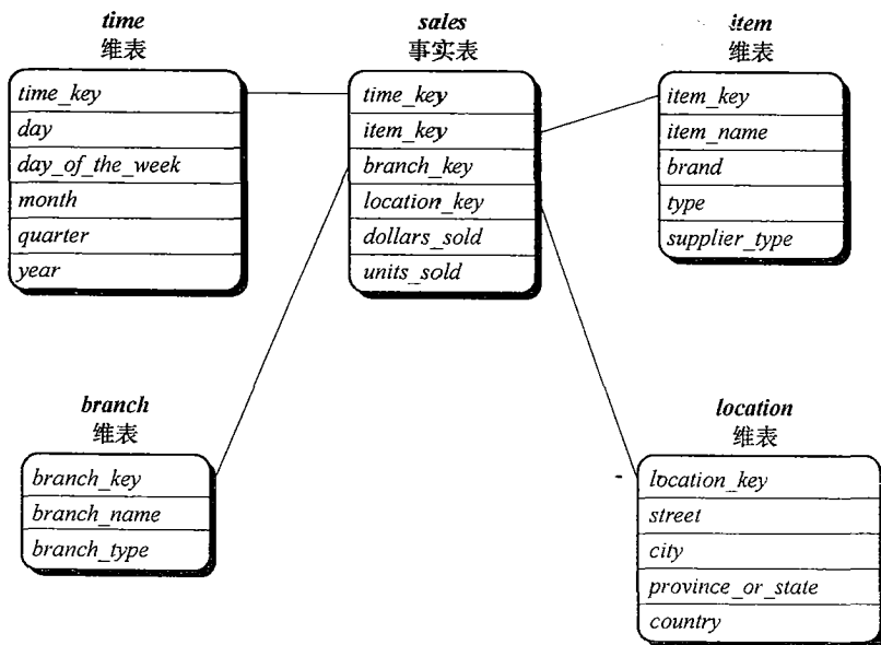
图 4.6 sales 数据仓库的星形模式
