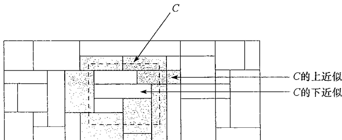
427 图 9.14 类 C 的元组集 (使用 C 的上、下近似集) 的粗糙集近似。矩形区域表示等价类
