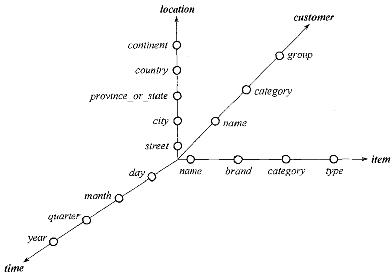
图 4.13 商务查询星网模型
