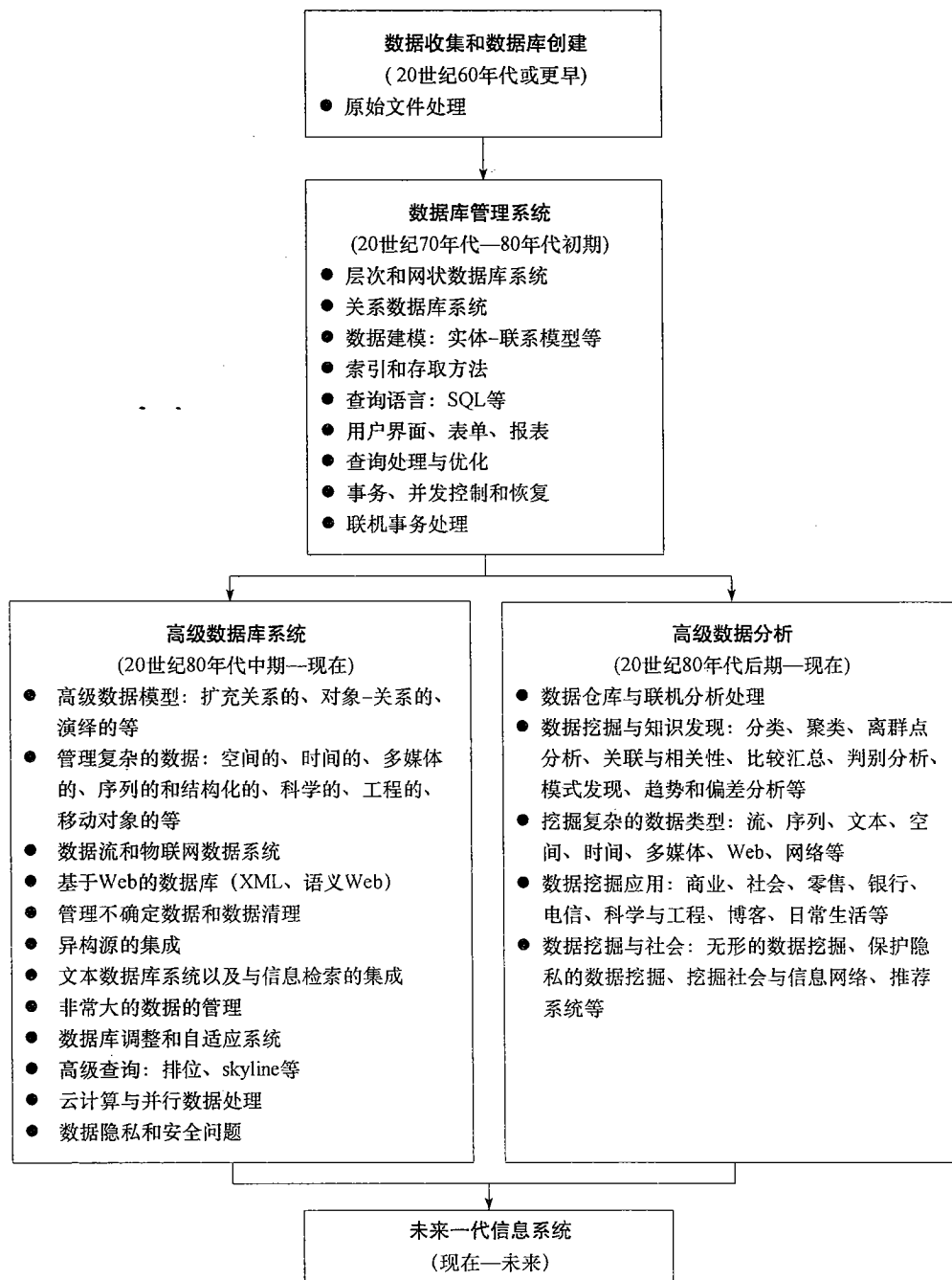
图 1.1 数据库系统技术的演变
