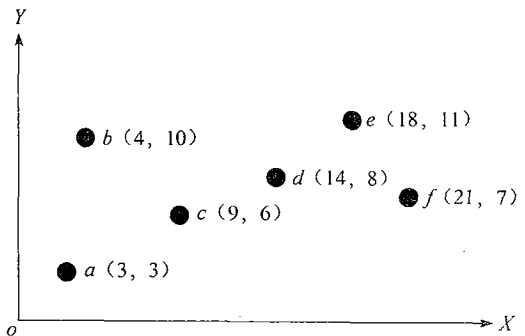
图 11.2 模糊聚类的数据集
