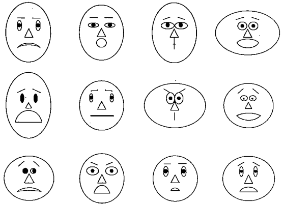
图 2.17 切尔诺夫脸。每张脸表示一个 n 维数据点 ( n \leq 18 )
