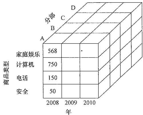
图 3.11 AllElectronics 的销售数据立方体
