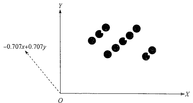
图 11.9 在导出的空间中聚类可能效果更好
