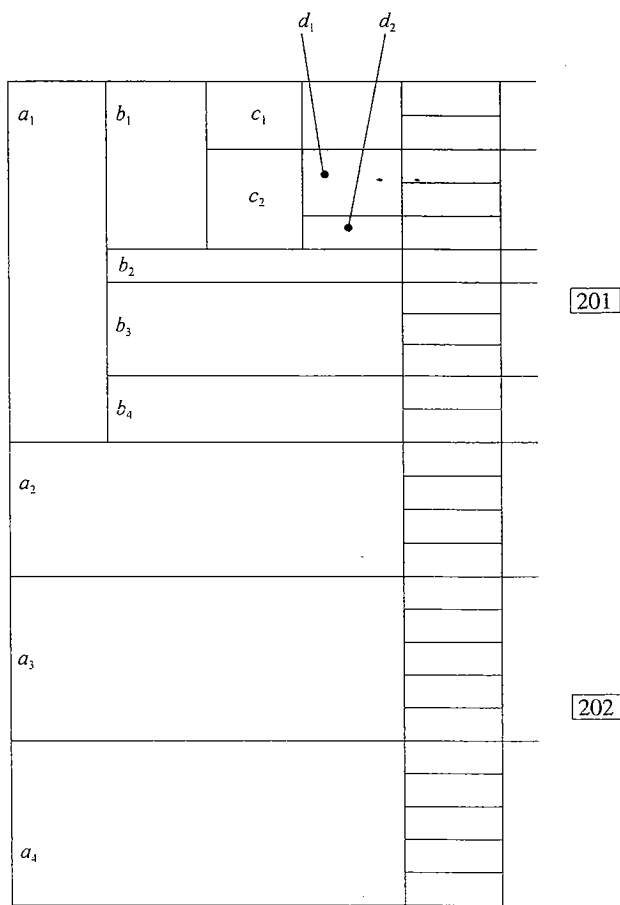
图 5.7 BUC 划分给定 4-D 数据集的快照
