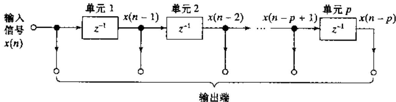
图 13-3 通常的 p 阶抽头延迟线记忆
