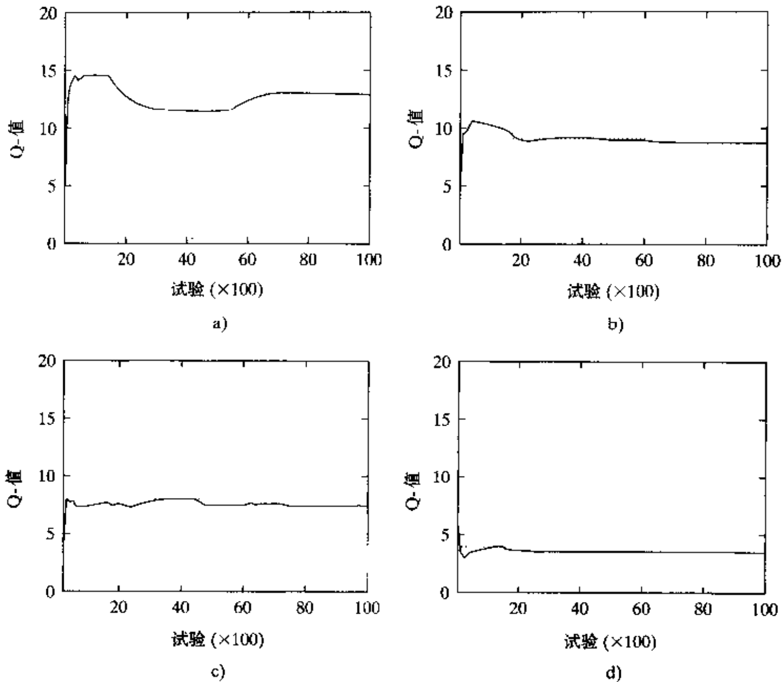
图 12-12 利用神经网络求解驿车问题的学习曲线
