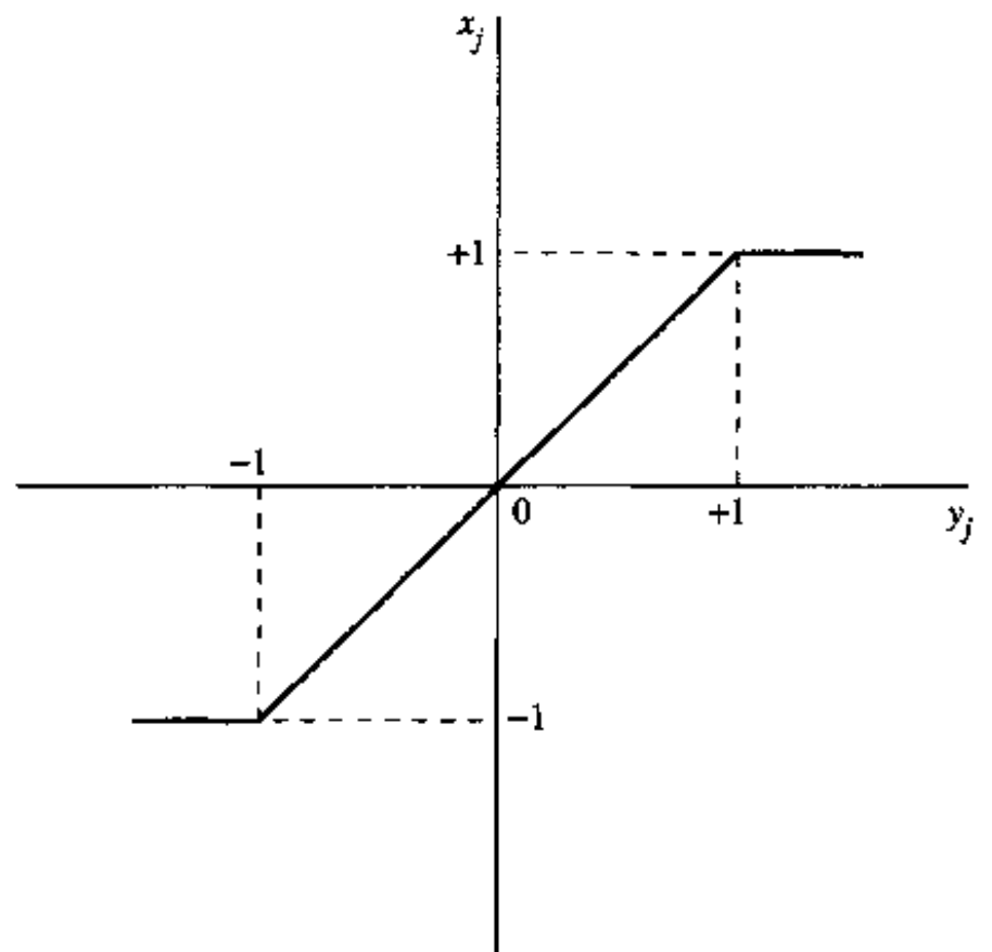
图 14-22 BSB 模型使用的分段线性函数
