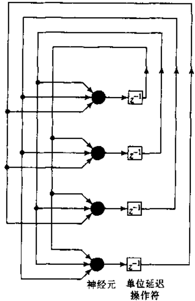
图 14-9 包含 4 个神经元的 Hopfield 网络结构图
