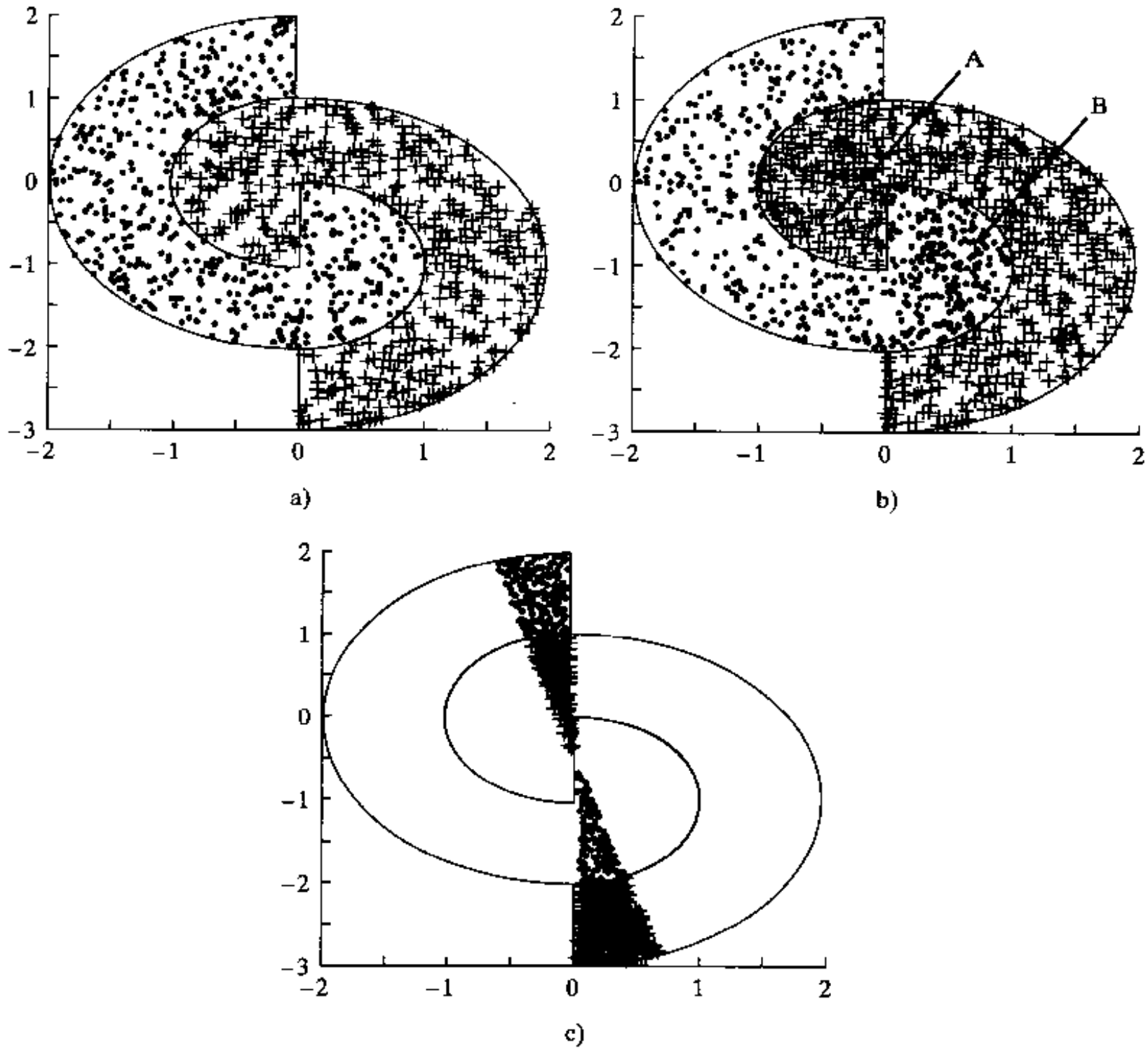
图 7-6 推举的计算机试验中用于专家训练的样本散布图
