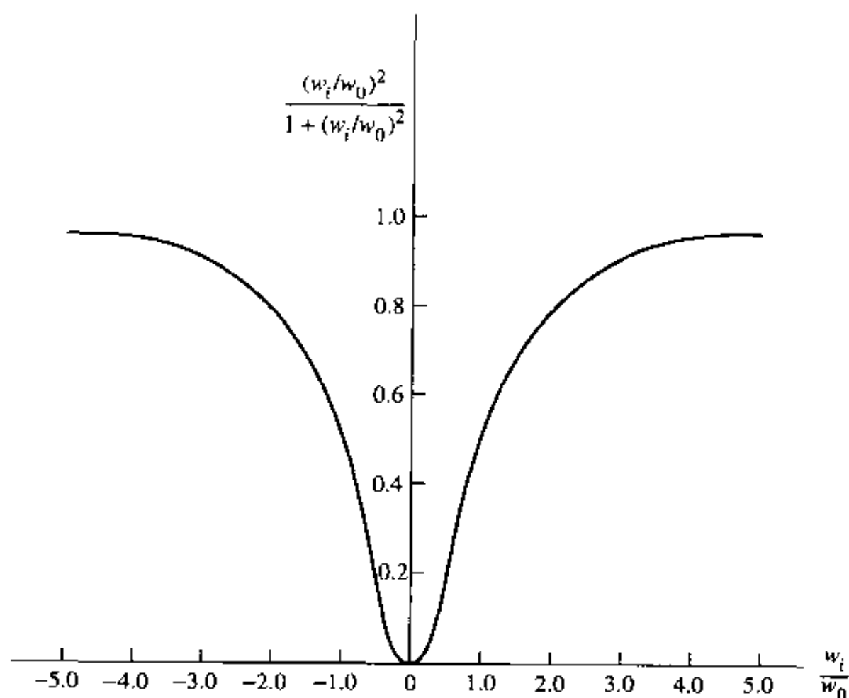
图 4-22 复杂性惩罚项 (w_i/w_0)^2/[1+(w_i/w_0)^2] 关于 w_i/w_0 的图示
