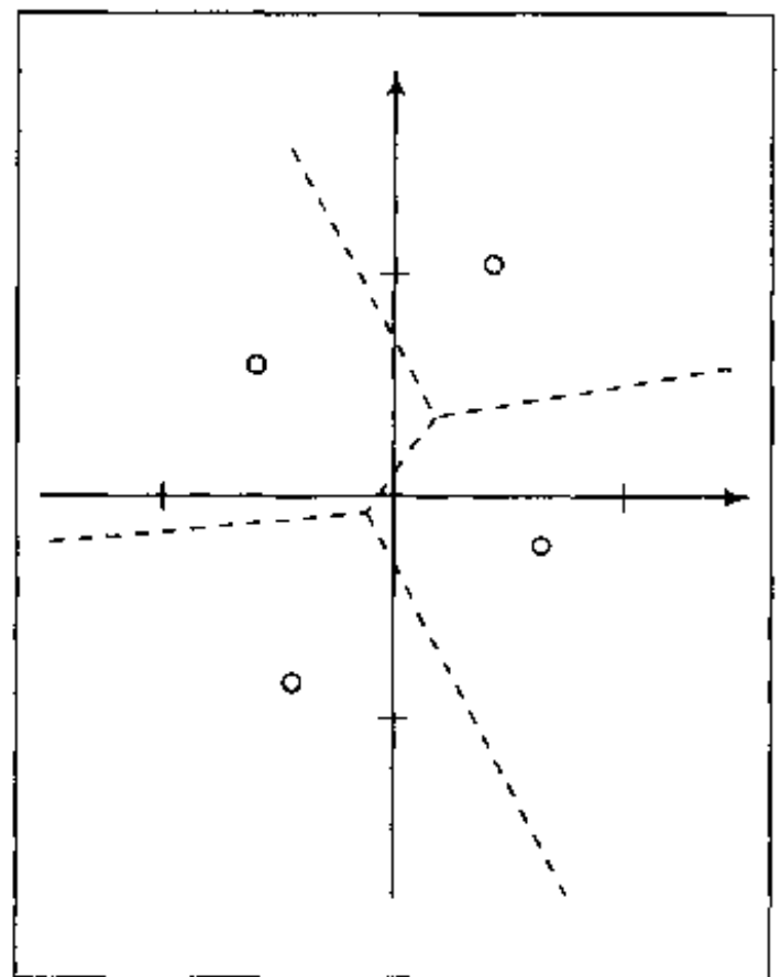
图 9-12 包含 4 个单元的 Voronoi 图 (经 IEEE 许可, 改自 R. M. Gray, 1984)
