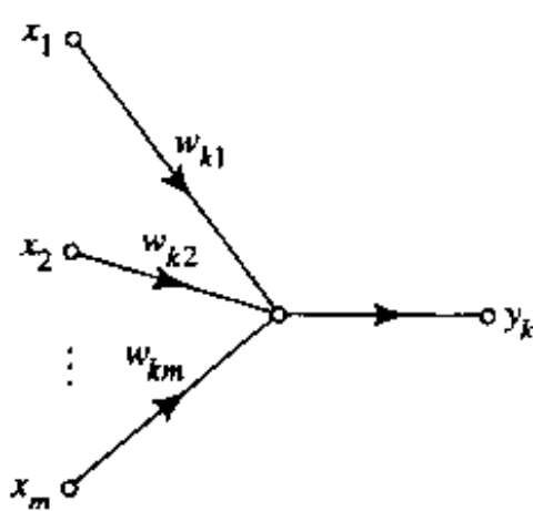
图 7-9 构成专家 k 的单个线性神经元的信号流图
