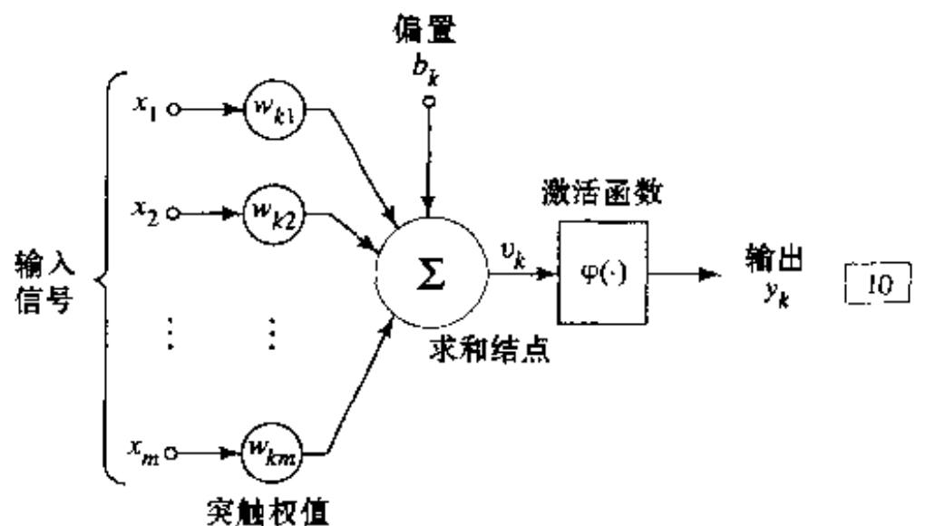
图 1-5 神经元的非线性模型
