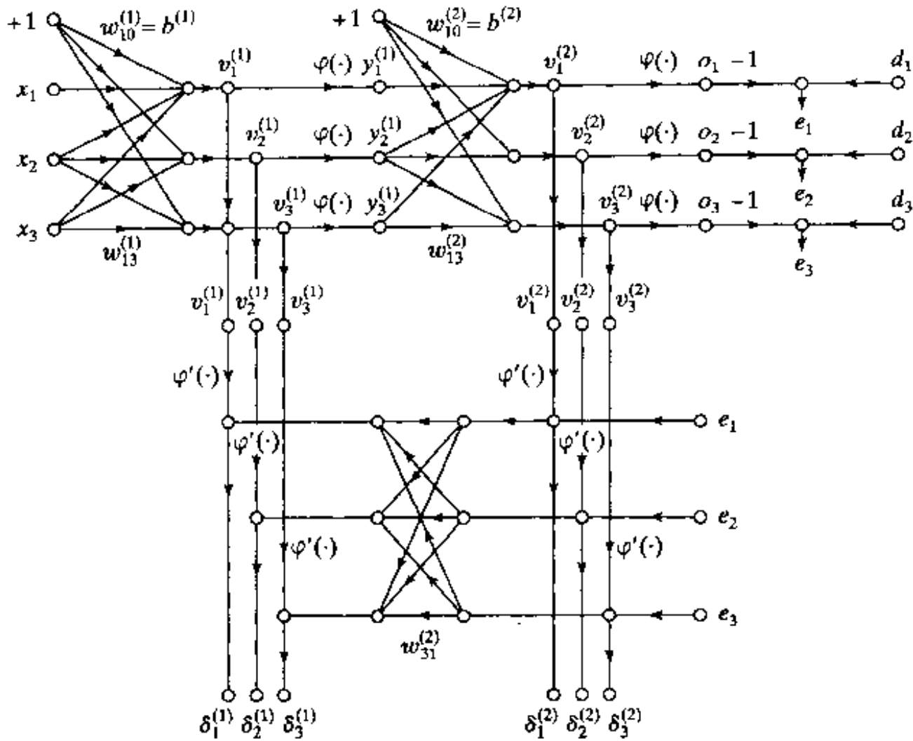
图 4-7 反向传播学习信号流图小结 图顶部：前向通过 图底部：反向通过
