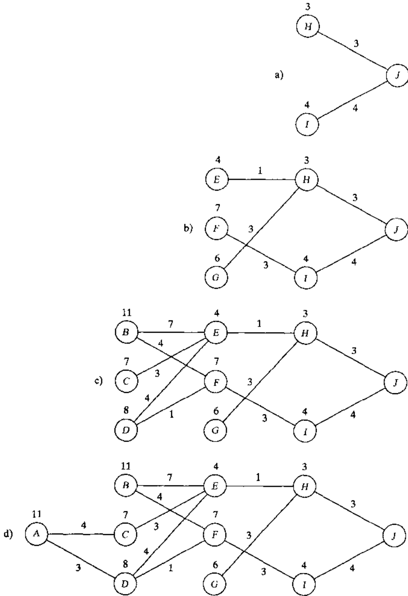
图 12-5 计算驿车问题 Q-因子涉及的步骤
