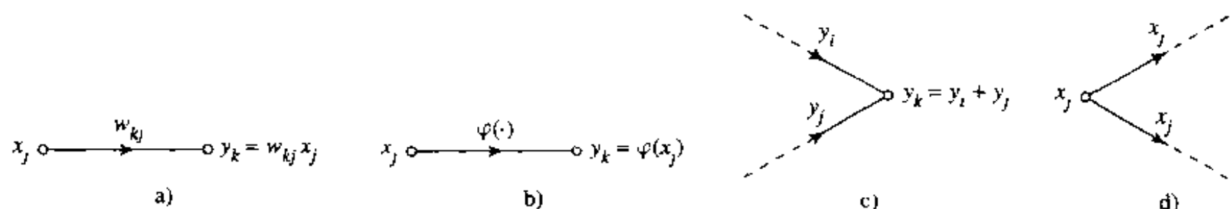
图 1-9 用于构造信号流图的基本规则图示
