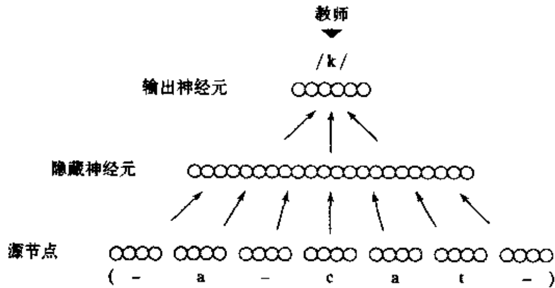
图 13-6 NETtalk 网络体系结构的示意图
