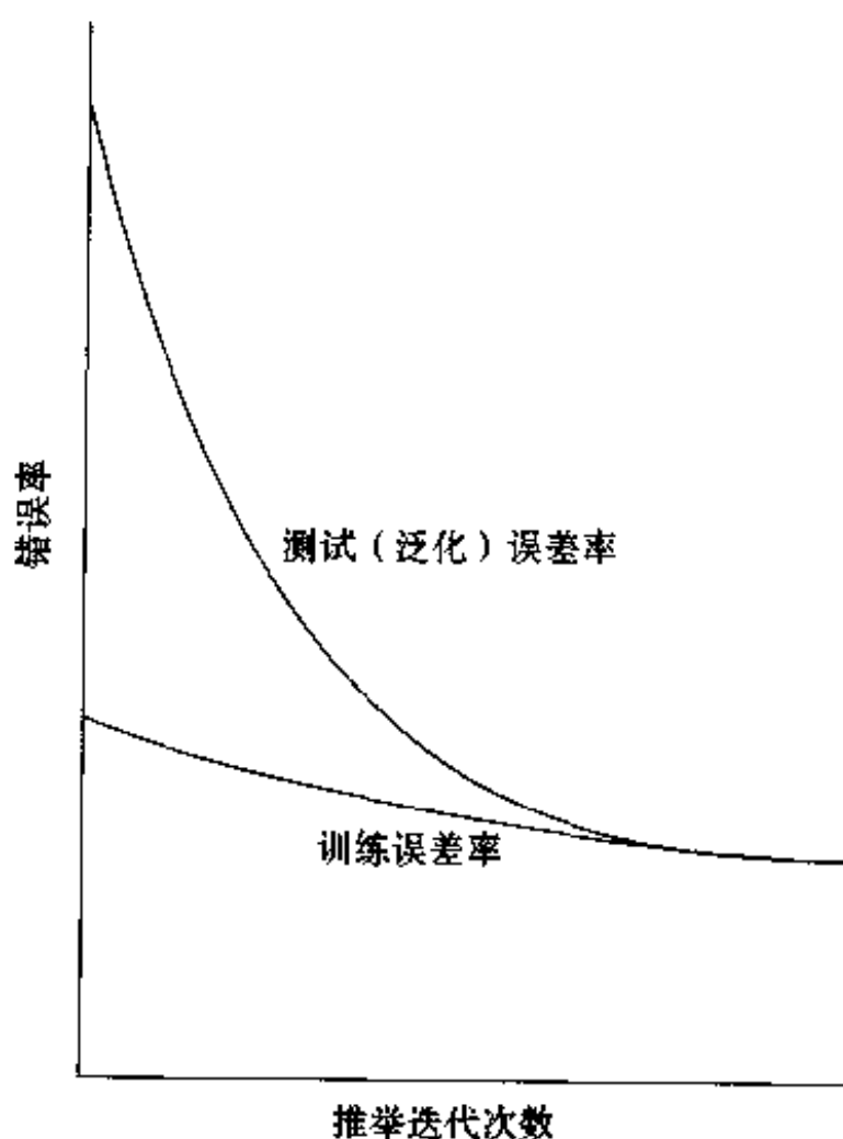
图 7-4 自举算法的概念化误差特性
