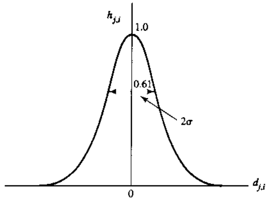
图 9-3 Gauss 邻域函数
