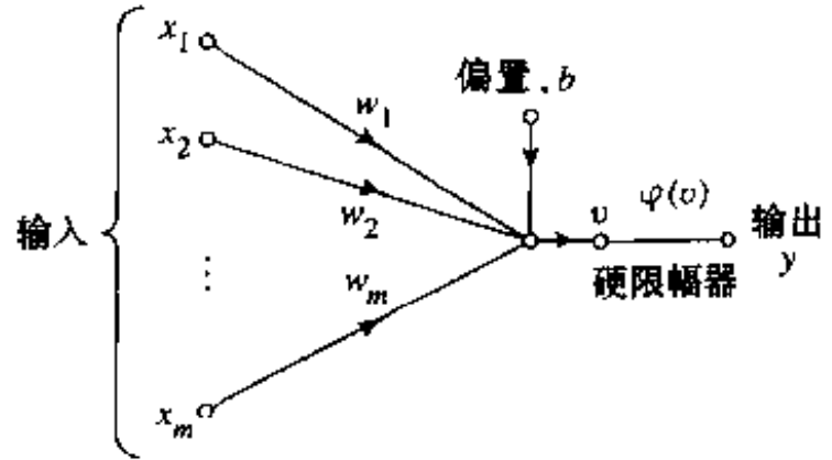
图 3-6 感知器的符号流图
