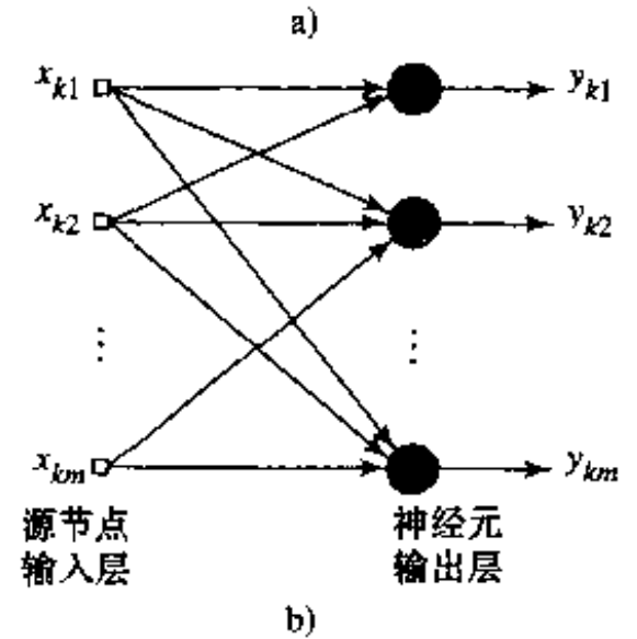
图 2-17 联想记忆模型
