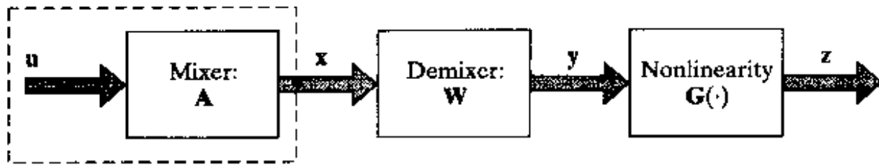
图 10-15 用于盲源分离的最大熵方法方框图 向量 \mathbf{u} , \mathbf{x} , \mathbf{y} 和 \mathbf{z} 分别是随机向量 \mathbf{U} , \mathbf{X} , \mathbf{Y} 和 \mathbf{Z} 的值
