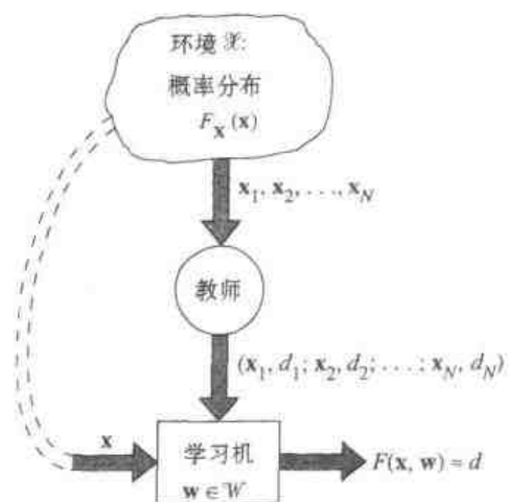
图 2-22 监督学习过程的模型
