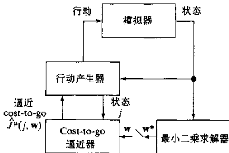
图 12-8 逼近策略迭代算法详细设计
