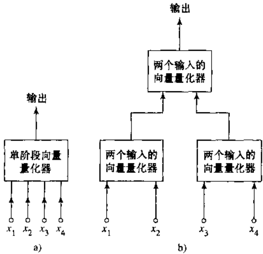
图 9-15 a) 具有四个输入的单阶段向量量化器 b) 使用两个输入的两阶段分层向量量化器 (摘自 S. P. Luttrell(1989a), British Crown 版权)
