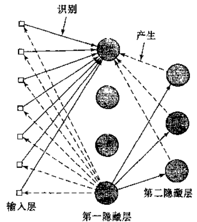
图 11-7 由识别(实线)连接和产生(虚线)连接的互连神经元构成的 Helmholtz 机结构图
