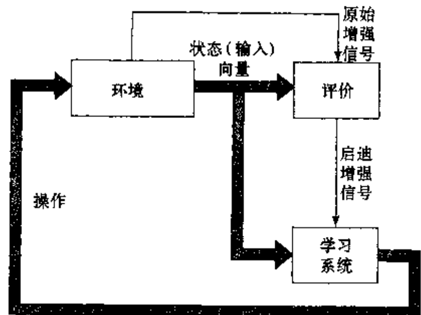
图 2-7 增强式学习方框图
