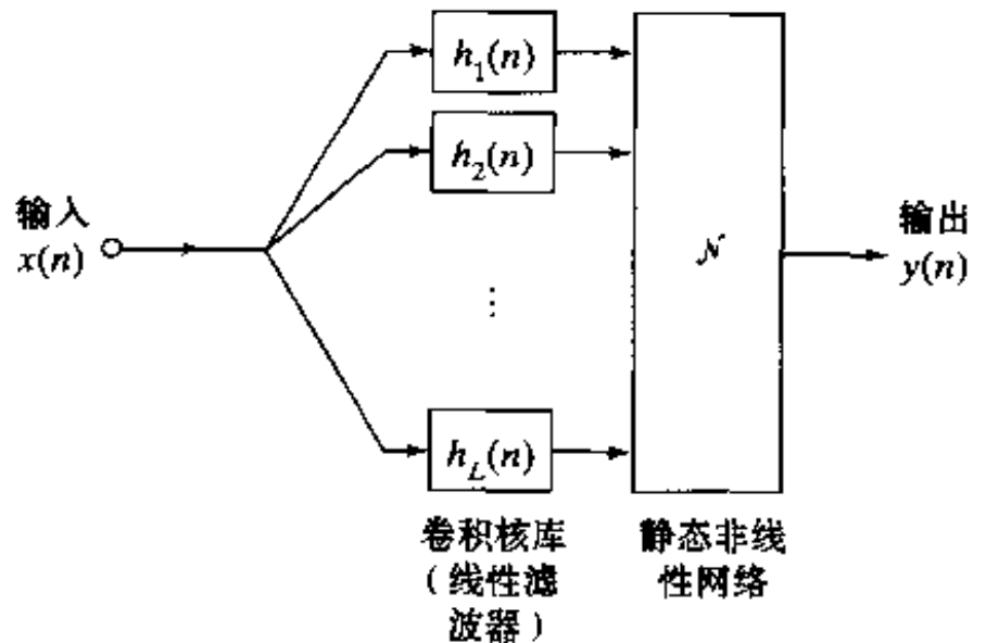
图 13-12 通用短视映射定理的一般结构
