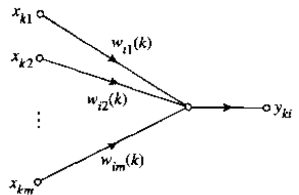
图 2-18 线性神经元 i 的信号流图模型
