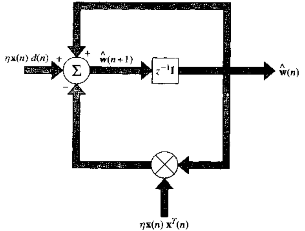
图 3-3 LMS 算法的信号流图表示
