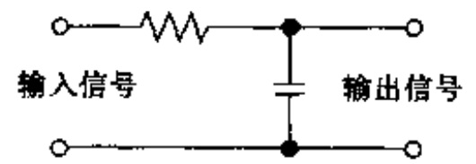
图 13-1 电阻电容电路
