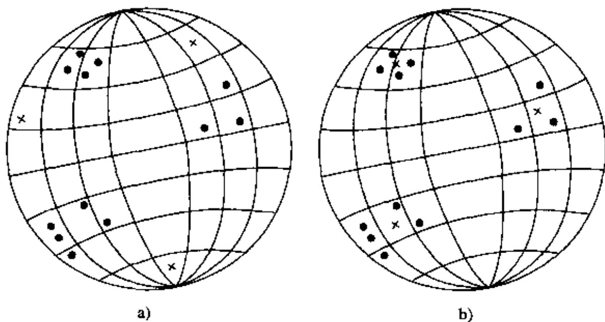
图 2-5 竞争学习过程的几何解释, 点代表输入向量, 叉代表 3 个输出神经元的突触权值向量 a) 网络的初始状态 b) 网络的终止状态
