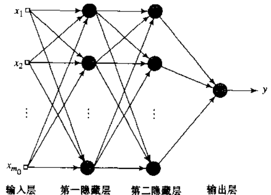
图 4-18 具有两个隐藏层和一个输出层的多层感知器
