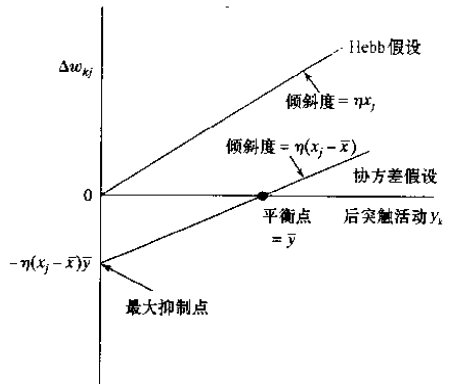
图 2-3 Hebb 假设和协方差假设的图示
