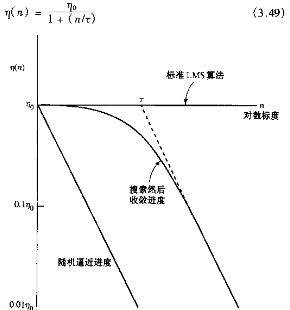
图 3-5 学习率退火进度
