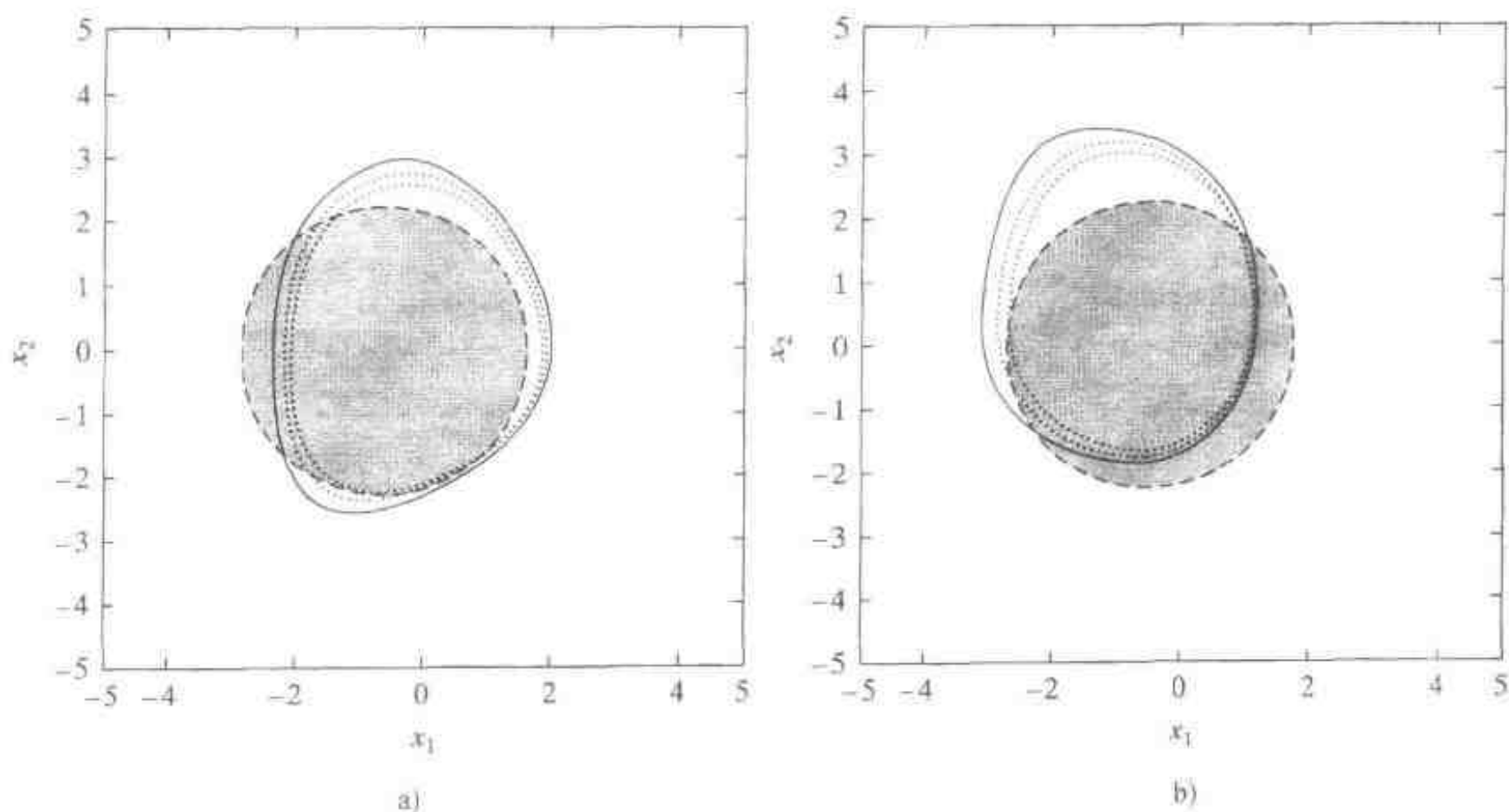
图 5-7 基于严格插值法的正则化 RBF 网络模式分类的试验结果
