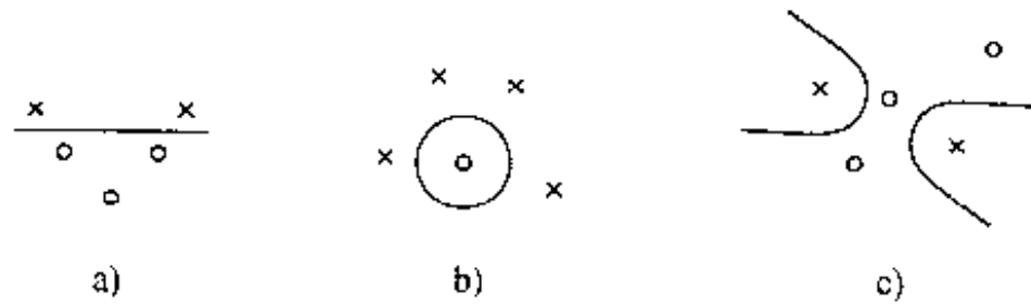
图 5-1 二维平面上的 5 个点的不同集合的 \varphi -可分的二分 3 个例子： a) 线性可分的二分 b) 球形可分的二分 c) 二次可分的二分
