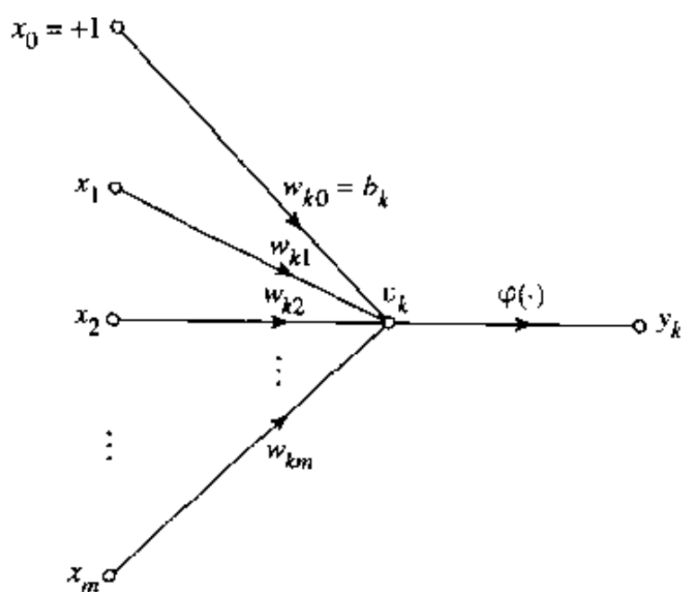
图 1-10 神经元的信号流图
