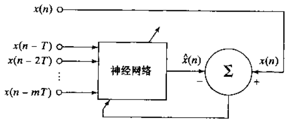
图 2-15 非线性预测方框图
