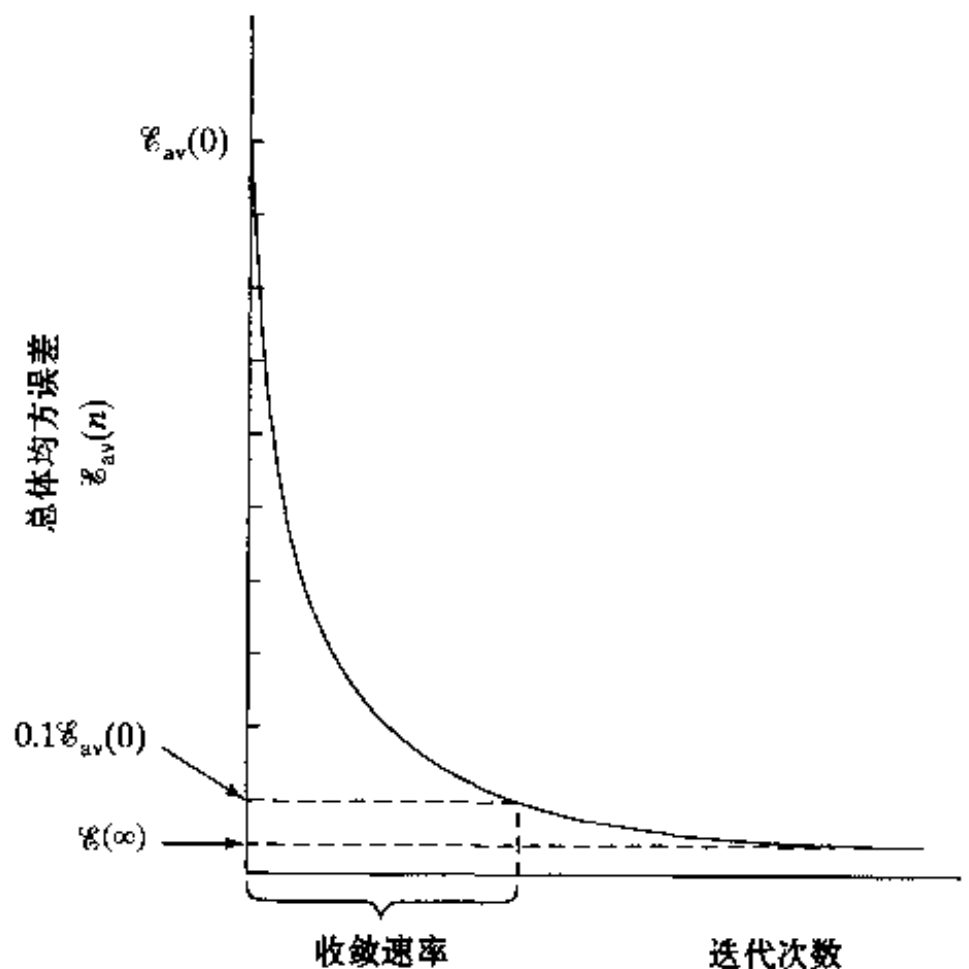
图 3-4 LMS 算法的理想学习曲线
