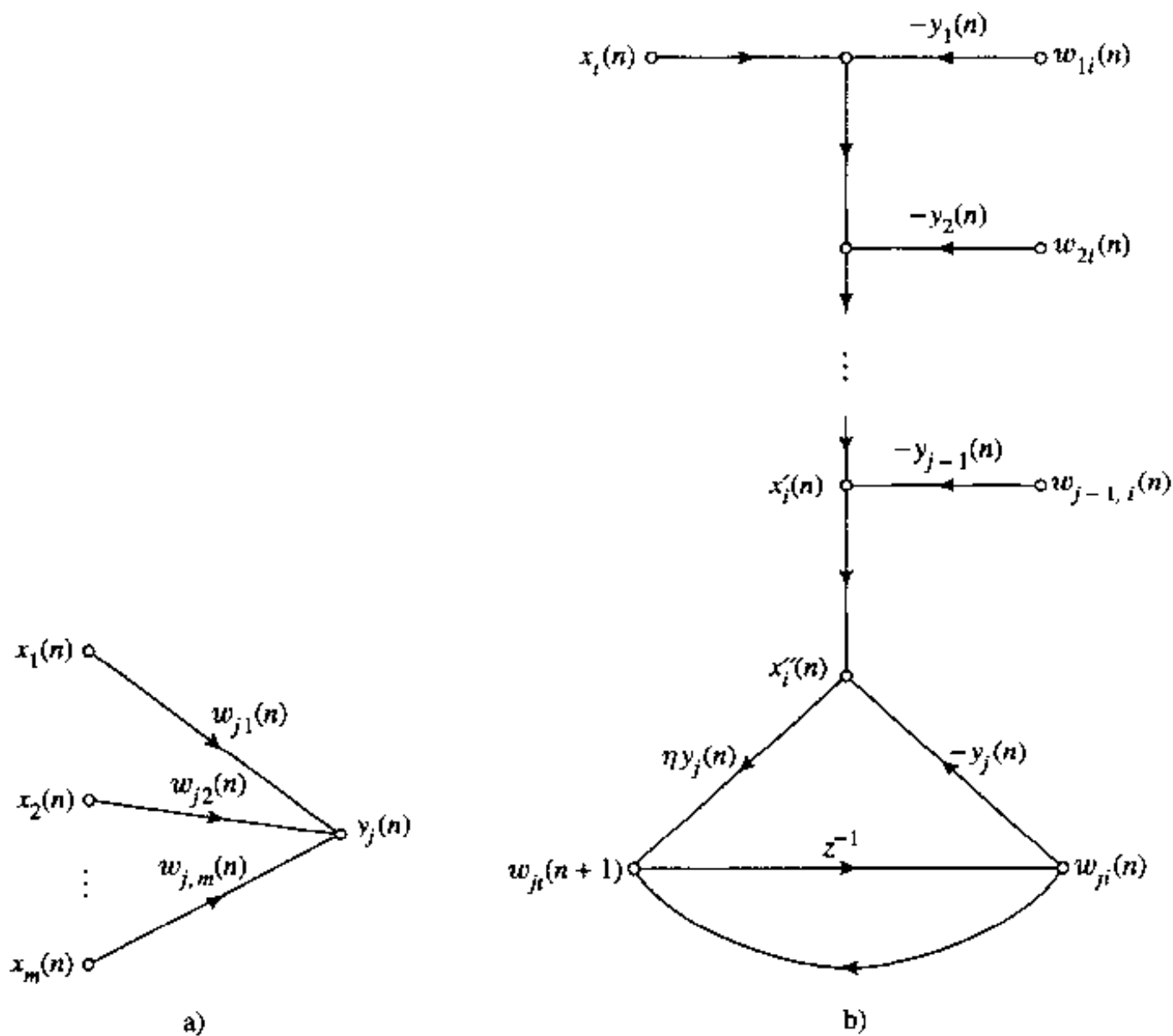
图 8-7 广义 Hebb 算法的信号流图表示 a) 式(8.79)的图 b) 式(8.80)至(8.81)的图
