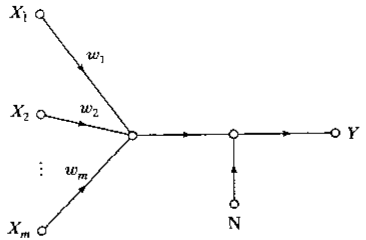
图 10-3 单个噪声神经元的信号流图
