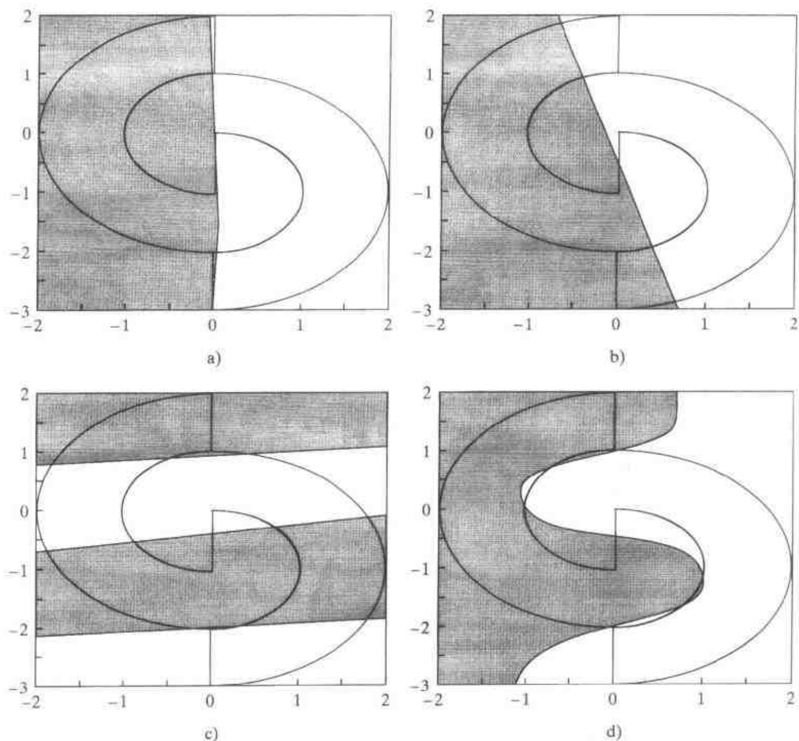
图 7-7 在推举试验中不同专家形成的决策边界 a)专家1 b)专家2 c)专家3 d)整个委员会机器
