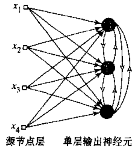
图 2-4 一个简单竞争学习网络的结构图, 它具有从源节点到神经元的前馈(兴奋的)连接和神经元之间的侧向(抑制的)连接(侧向连接由空心箭头标示出)
