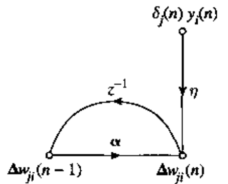
图 4-6 说明动量常数 \alpha 作用的信号流图
