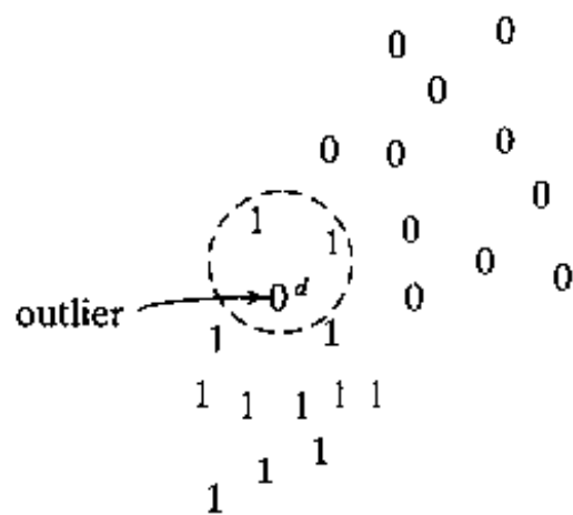
图 2-2 分类的例外
