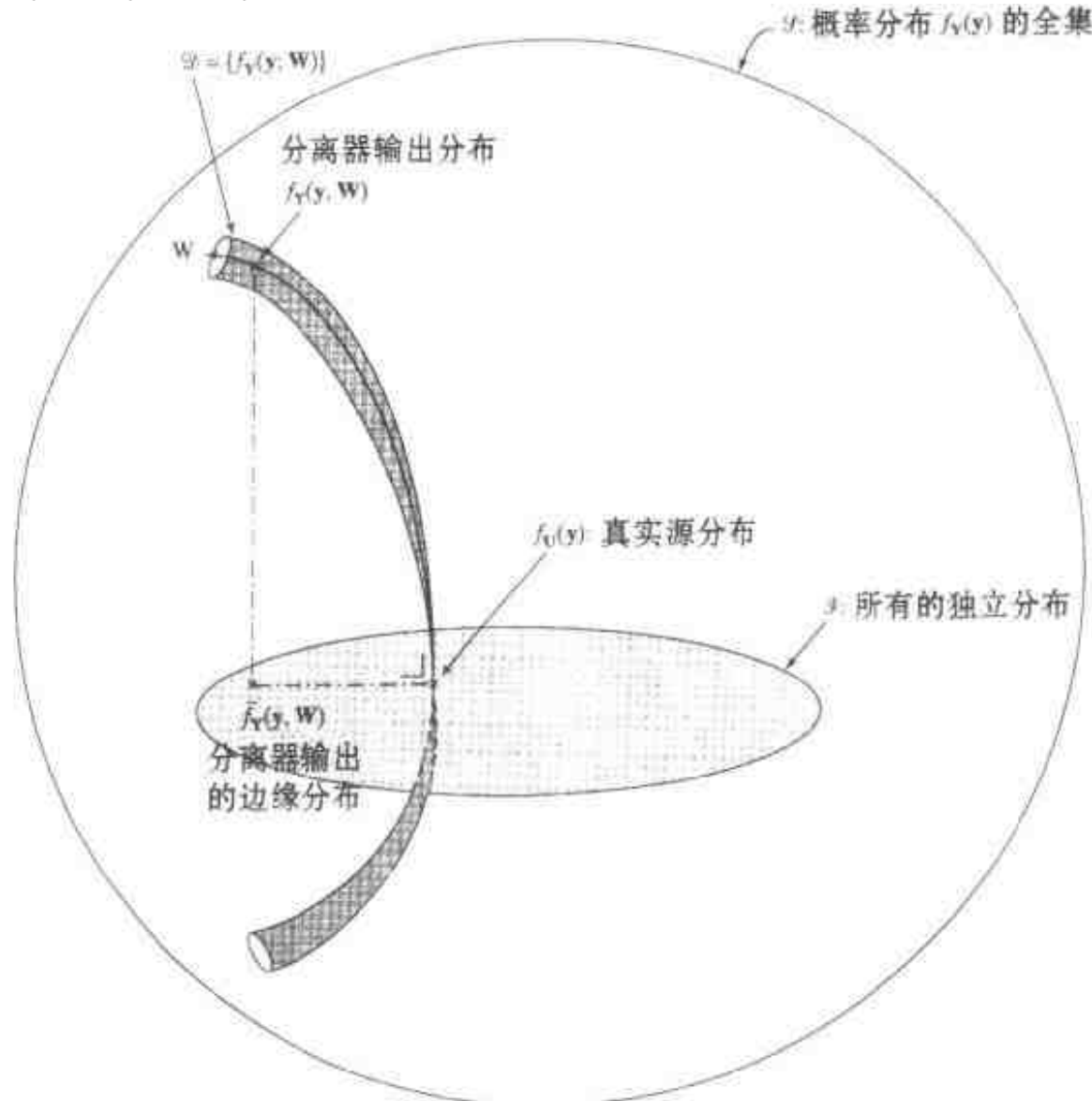
图 10-14 用于盲源分离的最大似然估计与独立分量分析之间的关系示意图 最大似然最小化 D_{f_Y \| f_U} ，而独立分量分析最小化 D_{f_Y \| \hat{f}_Y}
