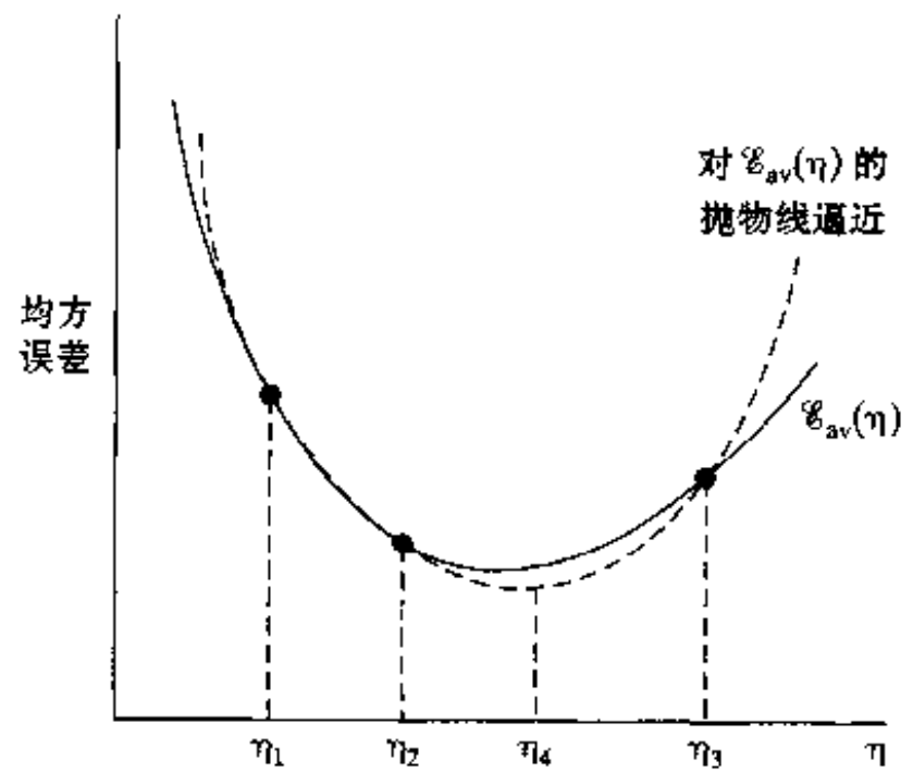
图 4-26 反抛物插值
