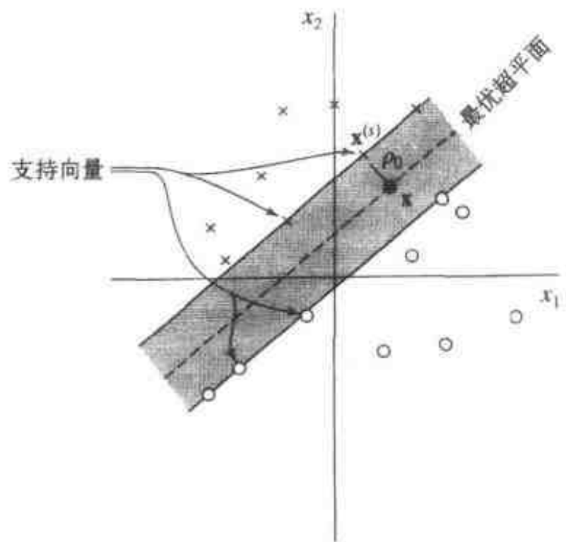
图6-1 线性可分模式最优超平面的思想示意图
