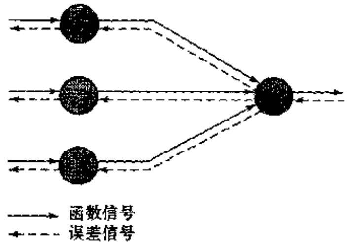
图 4-2 多层感知器中两个基本信号流的方向图示：函数信号的前向传播和误差信号的反向传播
