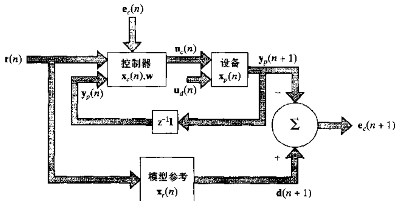
图 15-19 使用直接控制的模型参考自适应控制
