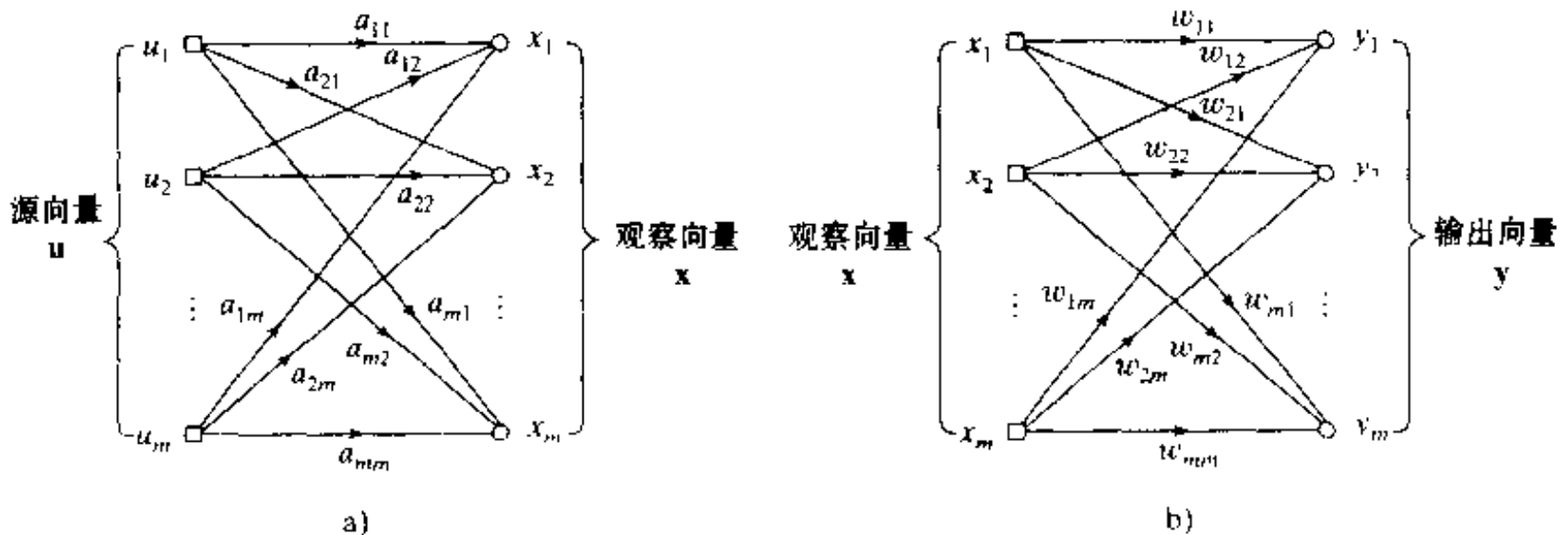
图 10-10 细节描述 a)混合矩阵 b)分离矩阵
