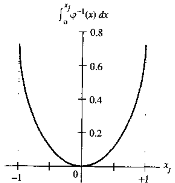
图 14-11 积分 \int_0^{x_j} \varphi^{-1}(x) dx 的图形
