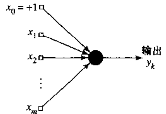
图 1-11 神经元的结构图
