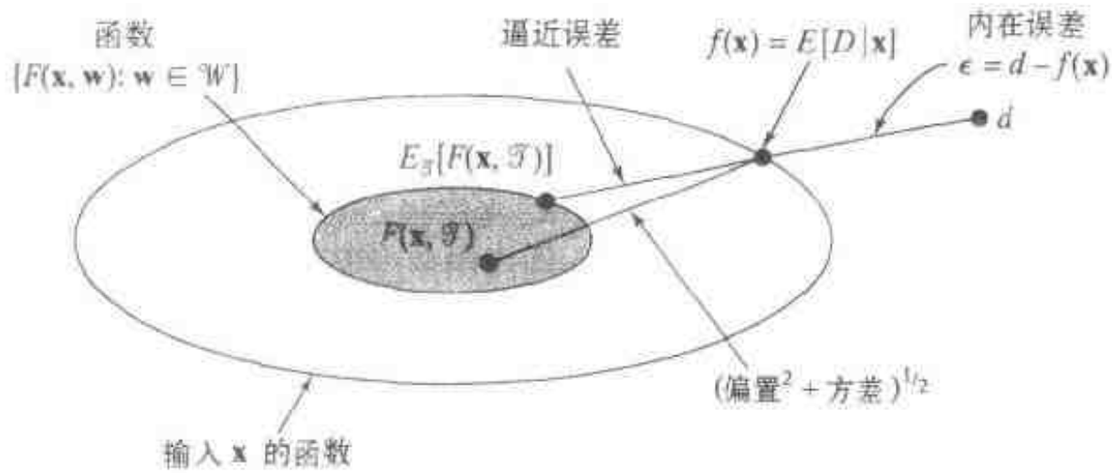
图 2-21 说明求解回归问题的各种误差源
