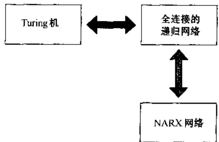
图 15-9 定理 I 和定理 II 及它们的推论的图解
