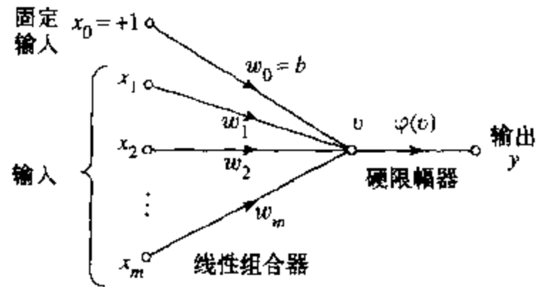
图 3-8 等价的感知器信号流图；为清楚起见省略了对时间的依赖性
