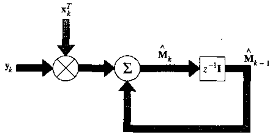
图 2-19 等式(2.38)的信号流图表示
