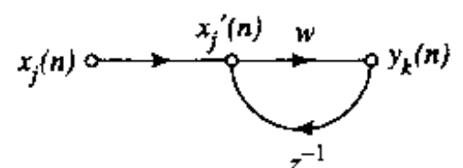
图 1-13 一阶无限冲击响应 (IIR) 滤波器的信号流图
