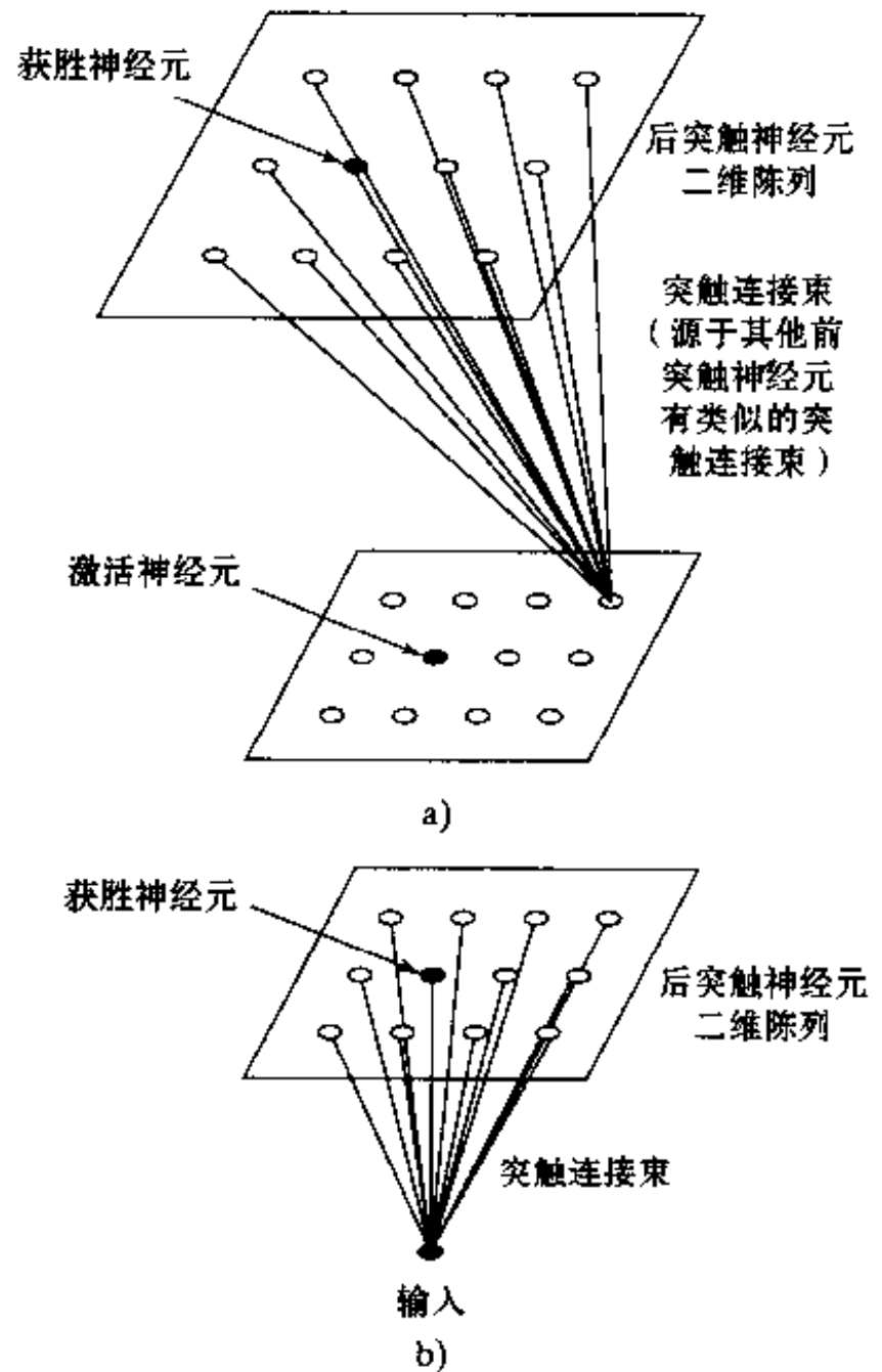
图 9-1 两个自组织特征映射 a) Willshaw-von der Malsburg 模型 b) Kohonen 模型
