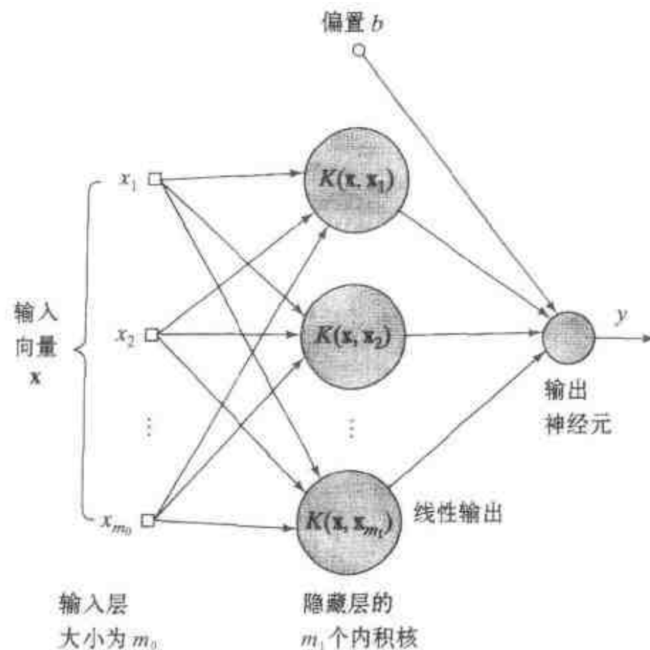
图 6-5 支持向量机的体系结构
