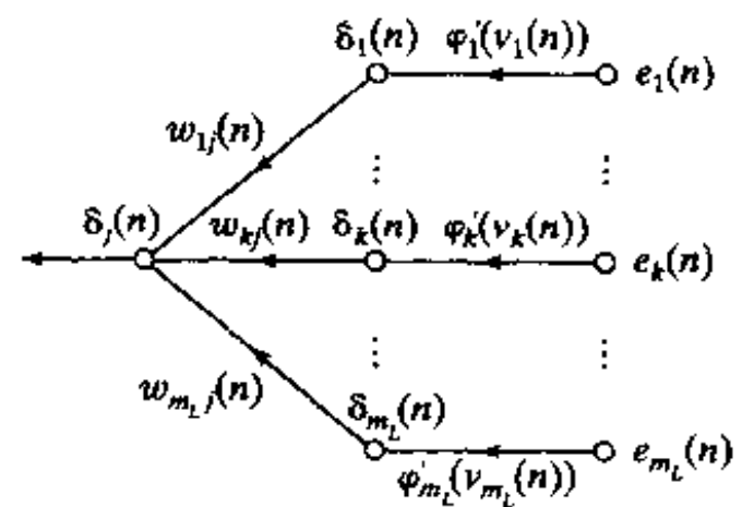
图 4-5 误差信号反向传播伴随系统的部分信号流图
