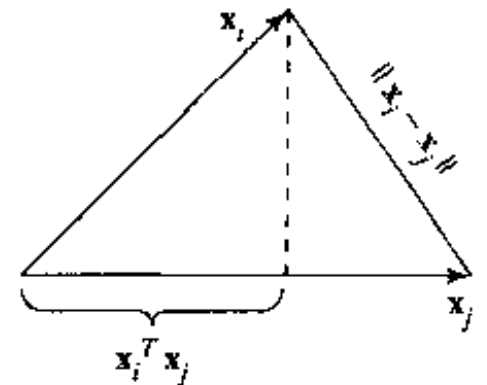
图 1-19 图解内积和作为模式相似性度量的欧几里德距离之间的关系
