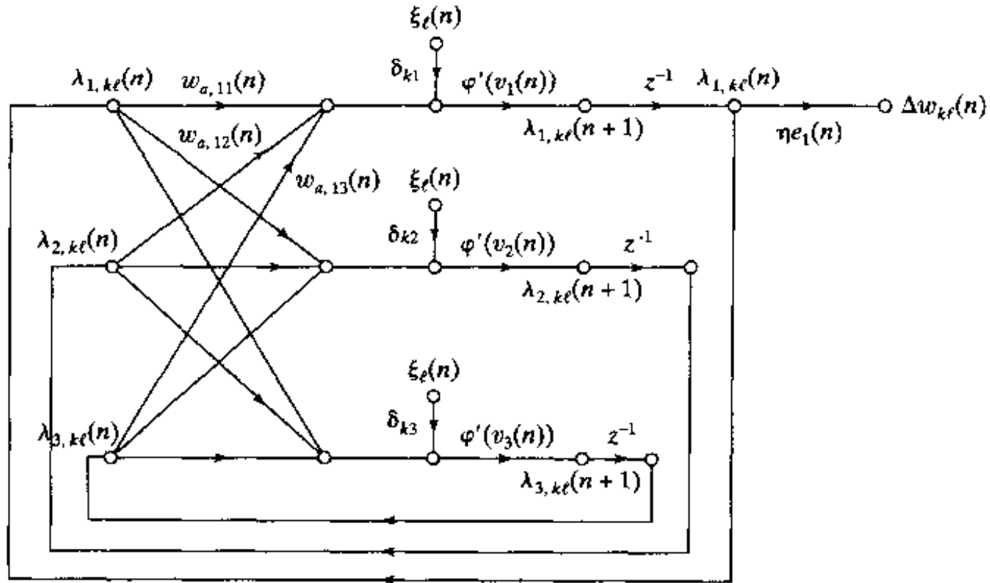
图 15-12 图 15-6 的全连接递归网络敏感度图 注意：标号为 \xi_i(n) 的三个节点都看作单输入
