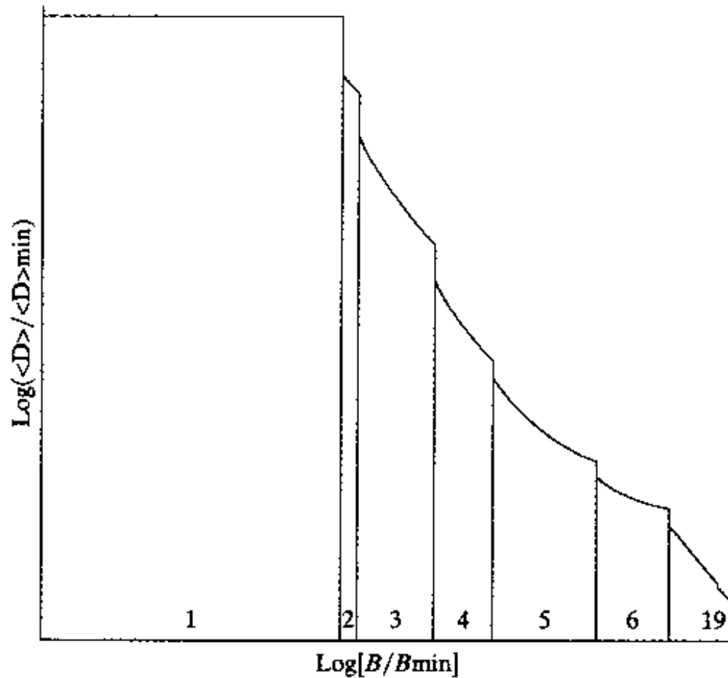
图 11-11 混合 Gauss 分布样本的相位图。对每个相位显示有效聚类的数目
