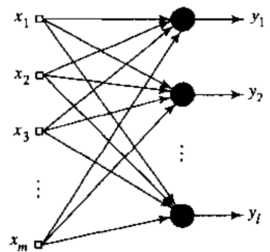
图 8-6 仅有单层计算节点的前馈网络
