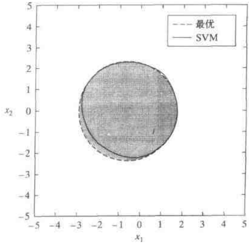
图 6-7 模式分类计算机实验的决策面
