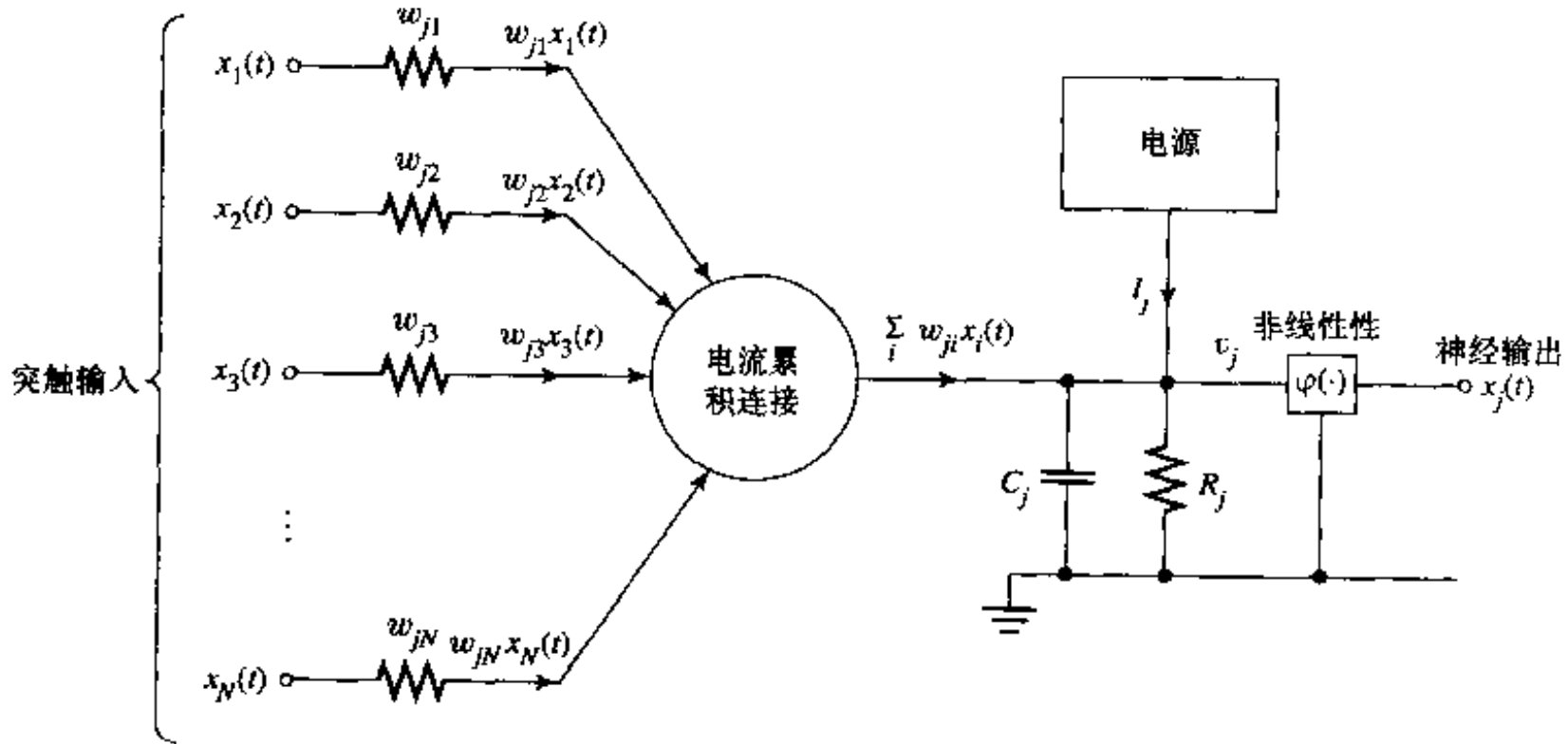
图 14-7 神经元的加性模型
