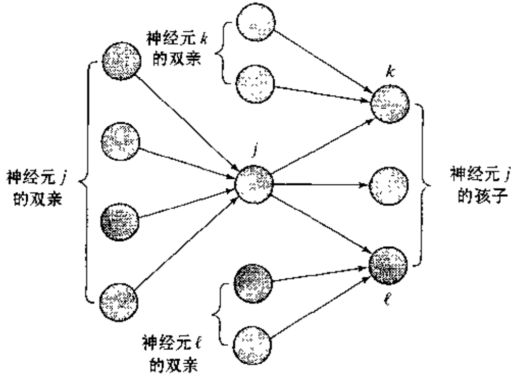
图 11-9 Markov 层举例
