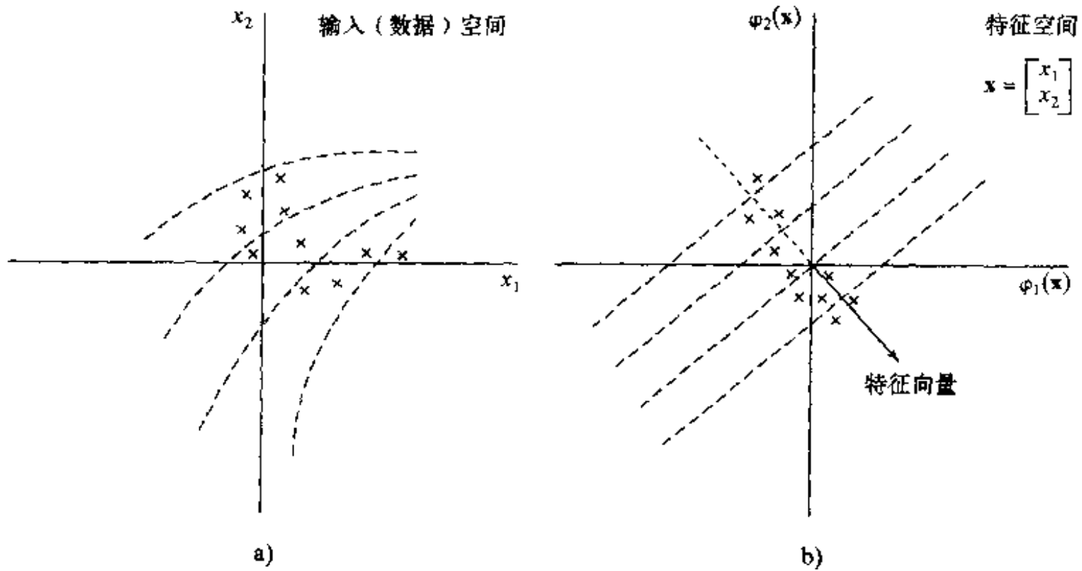
图 8-13 核 PCA 图例
