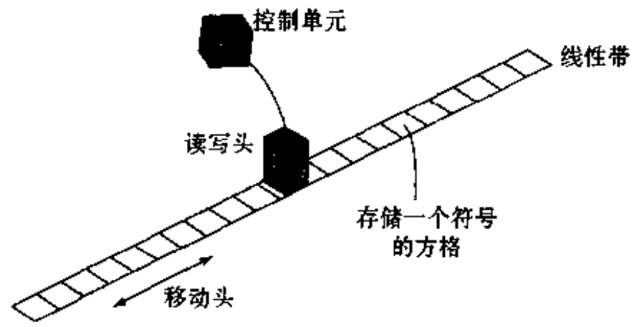
图 15-8 Turing 机
