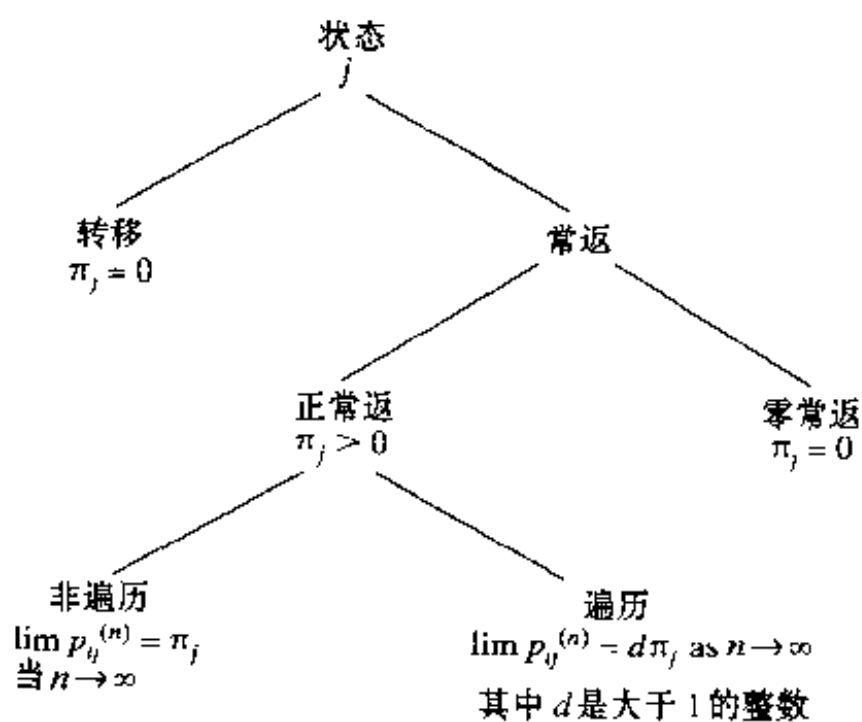
图 11-3 Markov 链的状态分类及它们相应的长期行为
