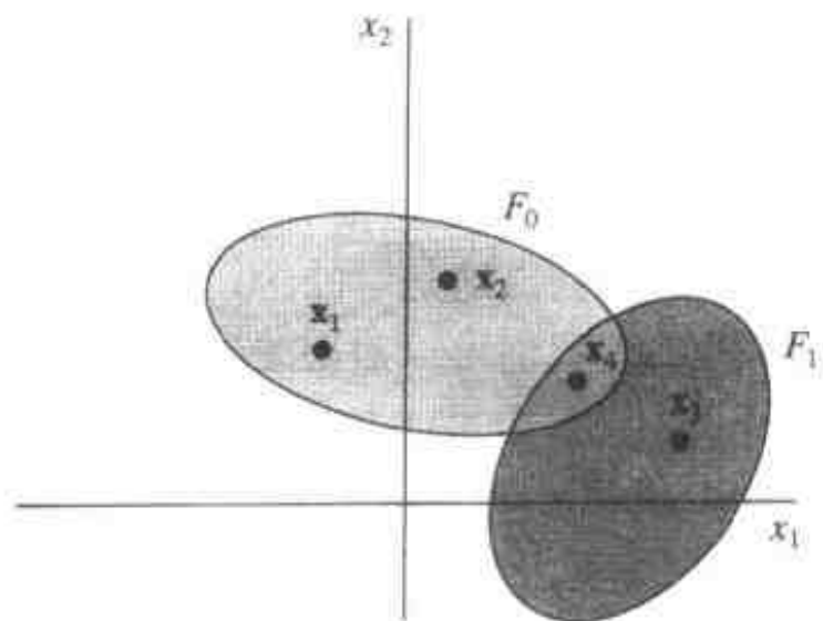
图 2-23 例 2-1 的图形
