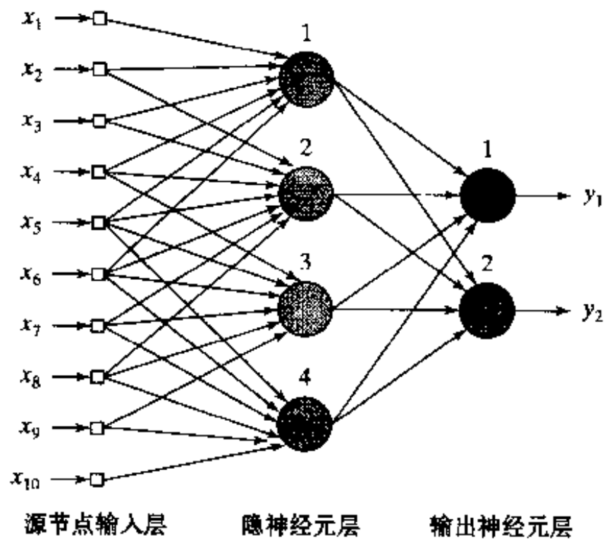
图 1-20 联合利用接受域和权值共享的图例。所有四个隐神经元共享它们突触连接的相同权值集
