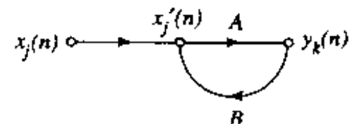
图 1-12 单环反馈系统的信号流图
